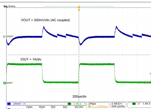
图 7-9. TPS542021EVM 负载瞬态响应, 0A 至 2A 负载阶跃
