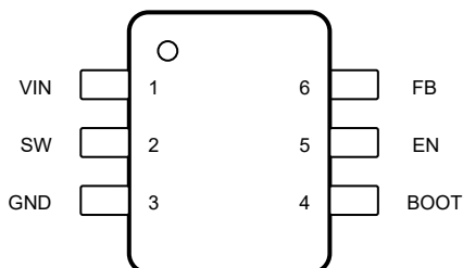
图 4-2. 6 引脚 SOT-563 DRL 封装 (俯视图)
