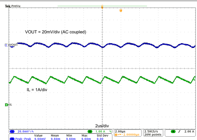
图 7-5. TPS542021EVM 输出电压纹波, I_{OUT} = 2A
