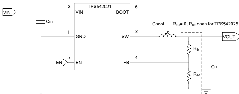
TPS54202x 简化原理图
