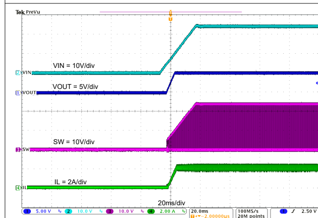
图 7-12. TPS542021EVM 相对于 V_{IN} 的启动
