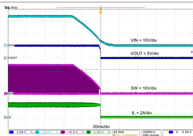
图 7-13. TPS542021EVM 相对于 V_{IN} 的关断
