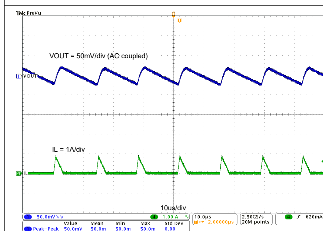
图 7-6. TPS542021EVM 输出电压纹波, I_{OUT} = 0.1A
