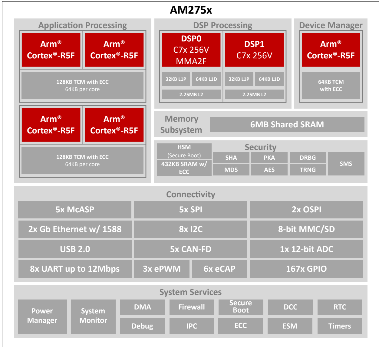
图 3-1. 功能方框图
