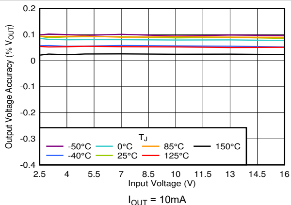
图 5-2. V_{OUT} 精度与 V_{IN} 间的关系
