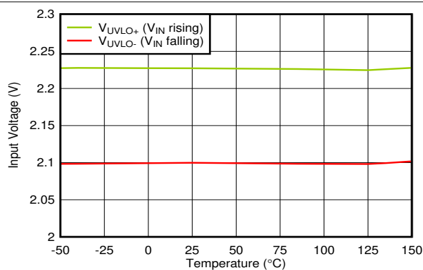
图 5-13. UVLO 阈值与温度间的关系
