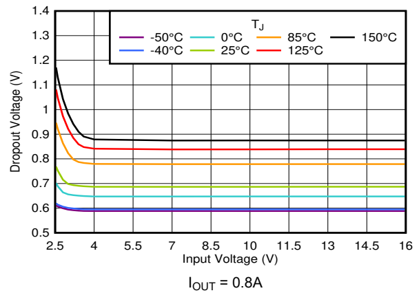
图 5-12. V_{DO} 与 V_{IN} 间的关系
