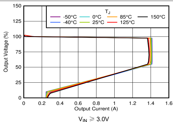
图 5-15. 折返电流限值与温度间的关系
