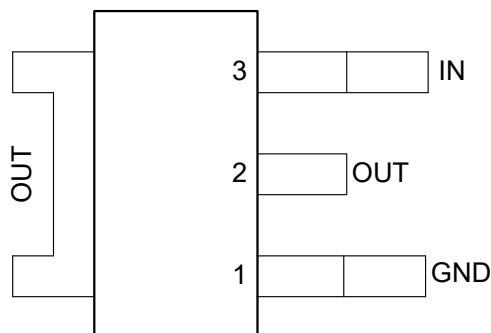
图 4-2. KVV 封装，3 引脚 TO-252 ( 顶视图 )
