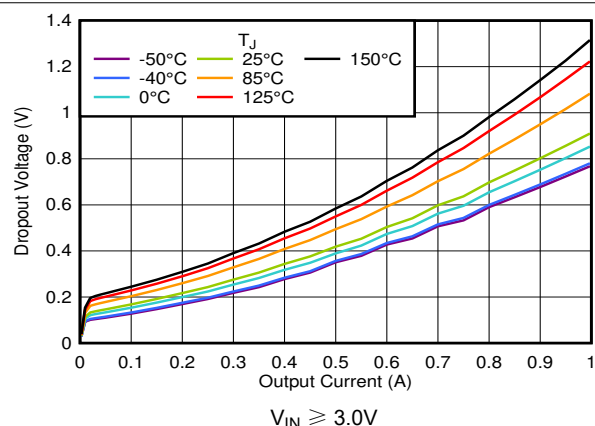
图 5-14. V_{DO} 与 I_{OUT} 间的关系
