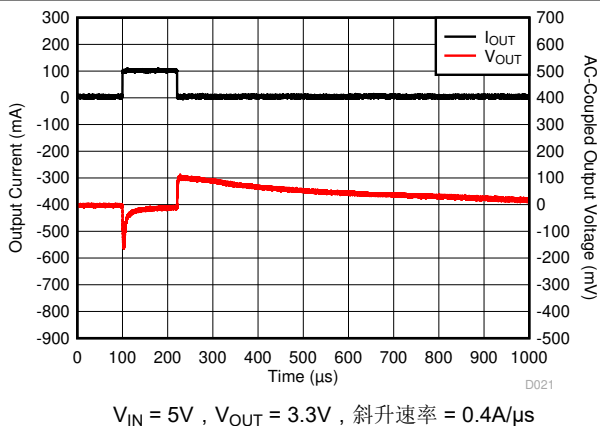
图 5-6. I_{OUT} 从 0mA 到 100mA 的瞬变
