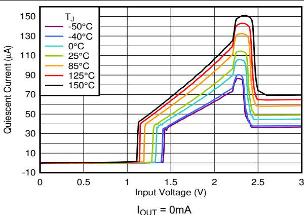
图 5-4. 当电压低于 V_{IN} 时 I_Q 会增加
