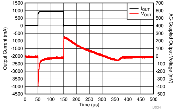
图 5-7. I_{OUT} 从 1mA 到 1A 的瞬变
