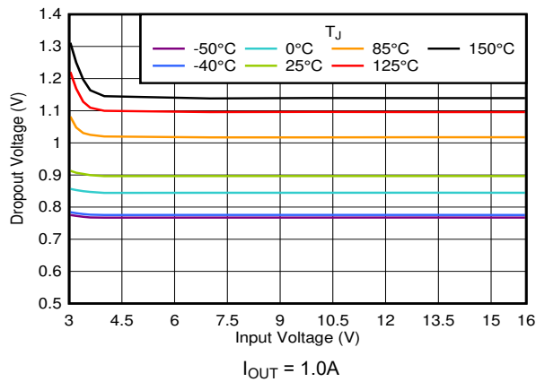
图 5-11. V_{DO} 与 V_{IN} 间的关系
