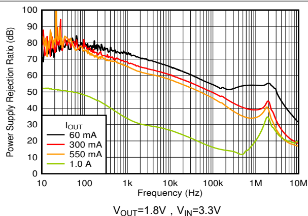
图 5-17. PSRR 与 I_{OUT} 间的关系
