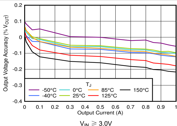
图 5-1. V_{OUT} 精度与 I_{OUT} 间的关系
