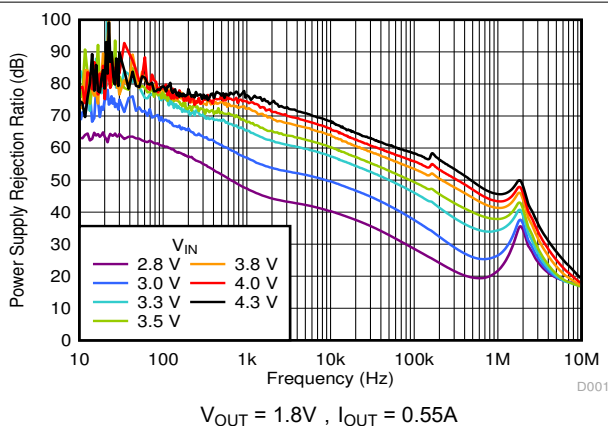
图 5-18. PSRR 与 V_{IN} 间的关系
