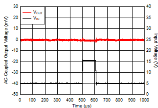
图 7-8. 从 5V 至 16V 的 V_{IN} 瞬态
