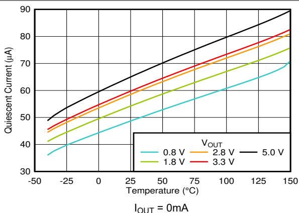
图 5-3. I_Q 与温度间的关系
