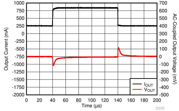
图 5-8. I_{OUT} 从 250mA 到 850mA 的瞬变
