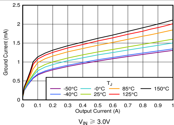
图 5-5. I_{GND} 与 I_{OUT} 间的关系
