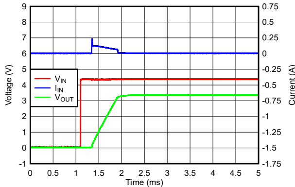
图 7-3. C_{OUT} 为 22 \mu\text{F} 时的启动和浪涌电流
