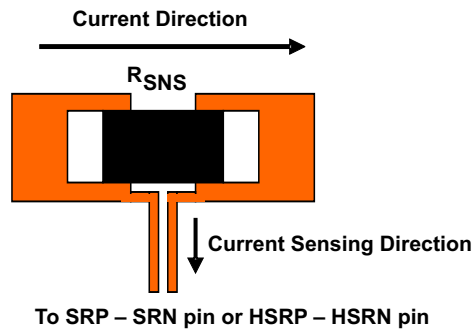
图 8-4. 检测电阻 PCB 布局
