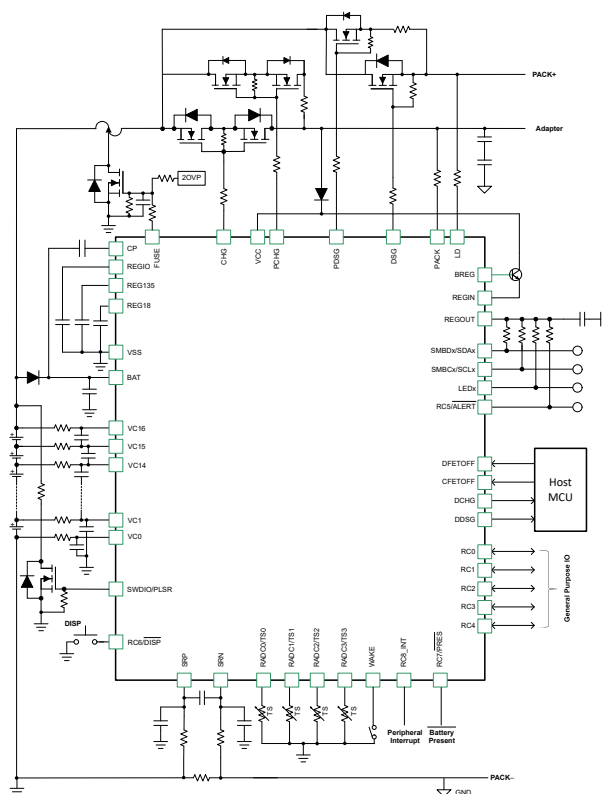
简化版原理图
