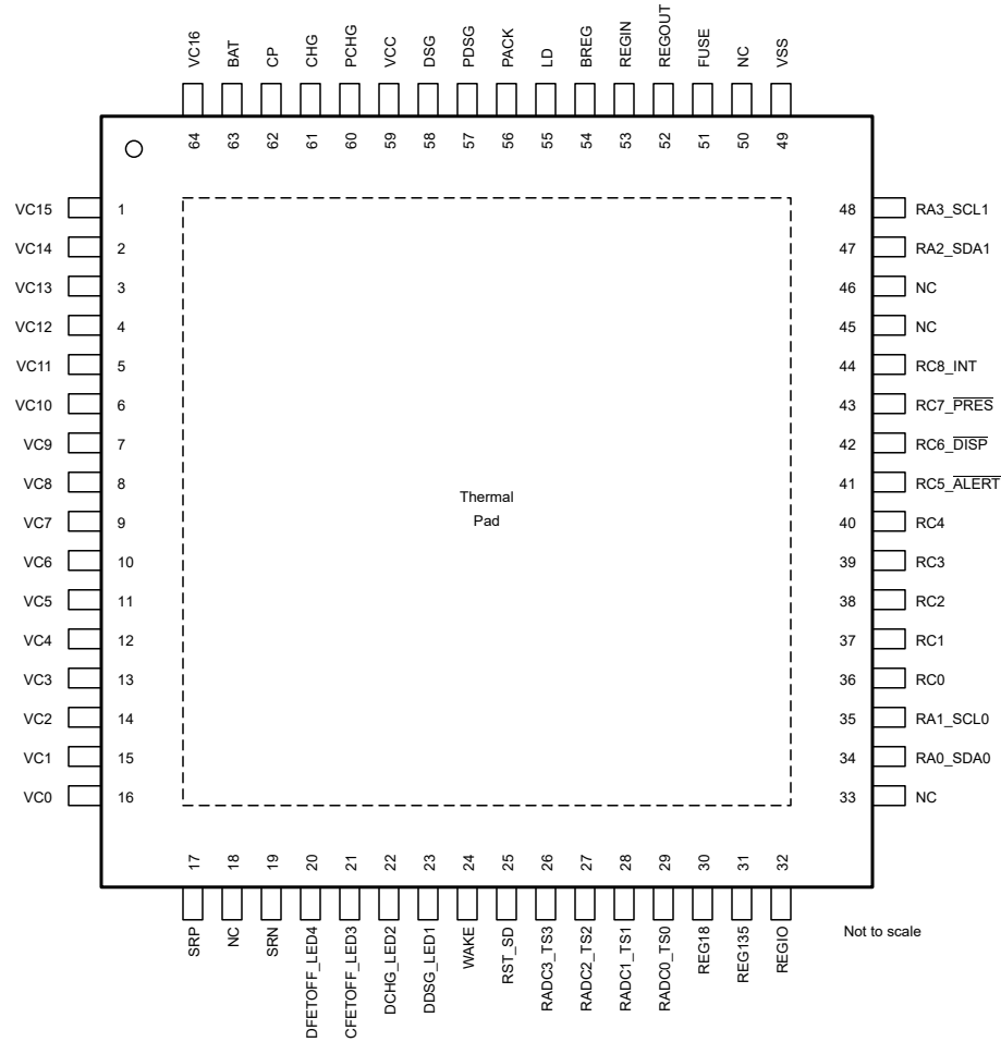
图 4-1. 引脚图
