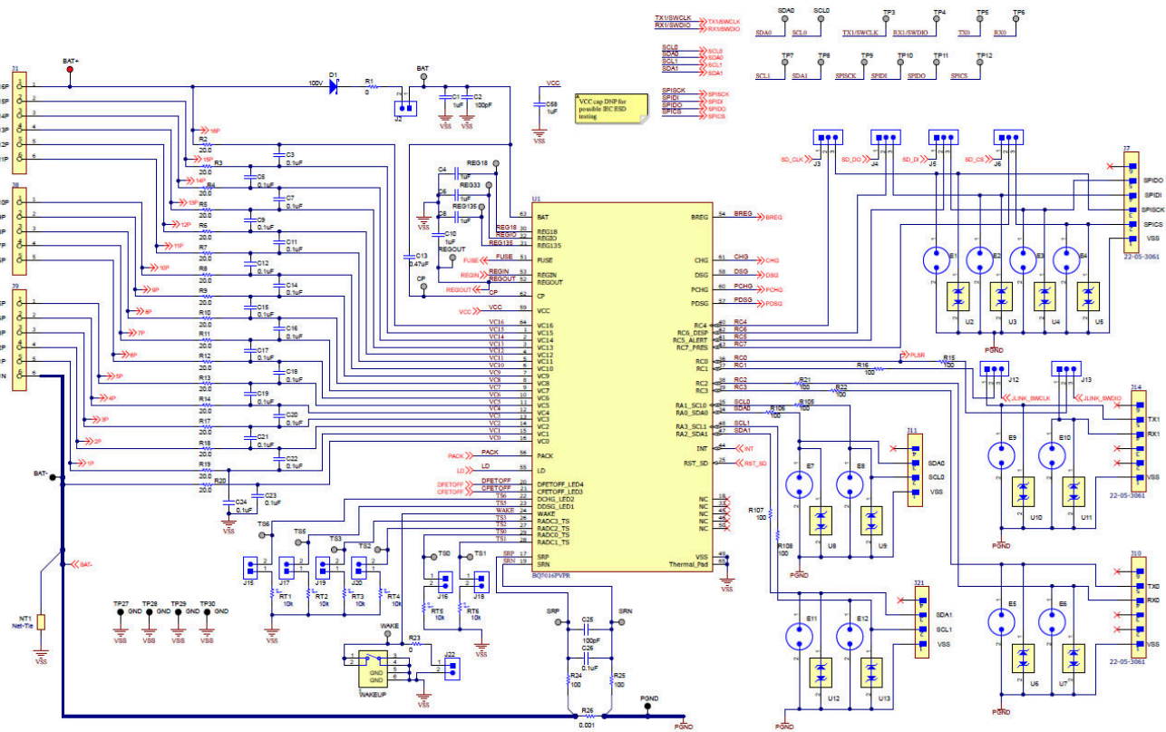
图 8-1. 典型应用
