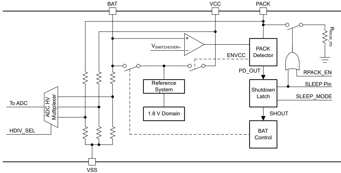
图 5-3. 电源引脚
