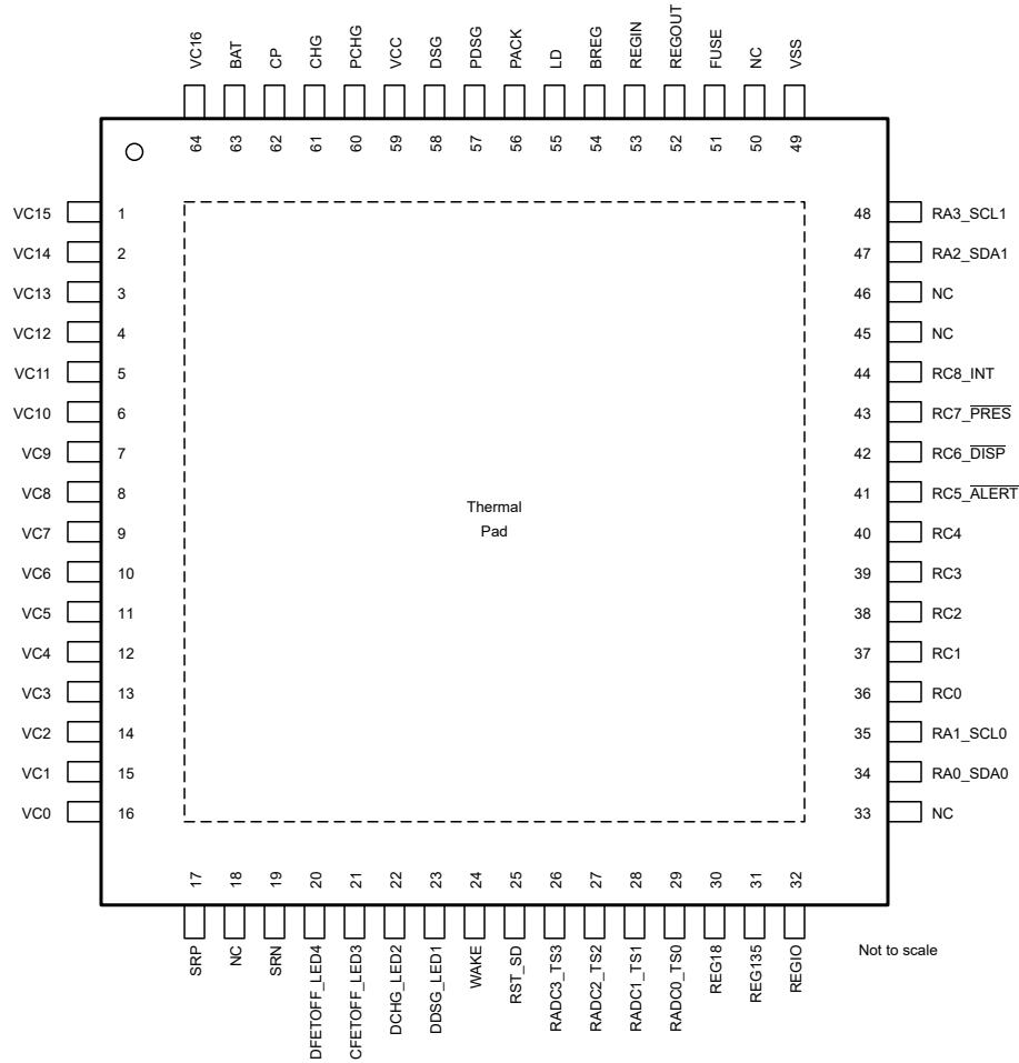
图 4-1. 引脚图
