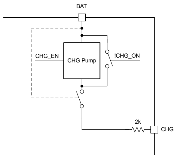
图 5-5. CHG 引脚
