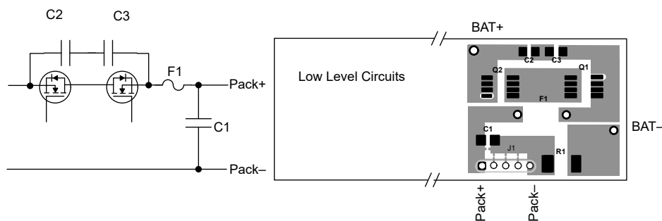
图 8-6. 使用宽覆铜布线降低旁路电容器 C1、C2 和 C3 的电感
