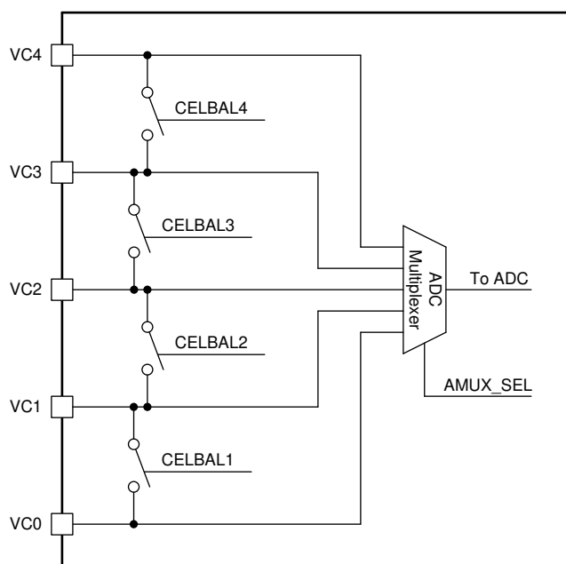
图 5-2. VCx 引脚
