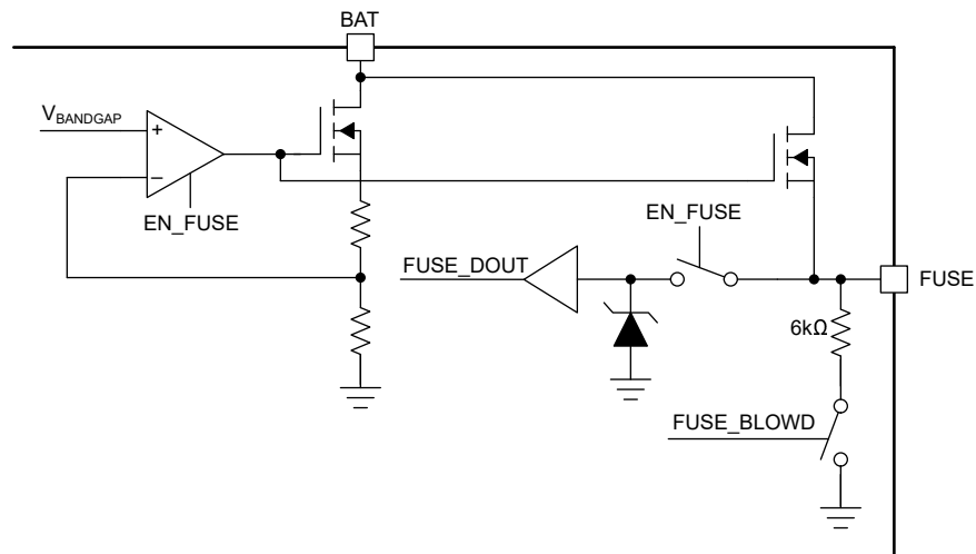
图 5-4. FUSE 引脚
