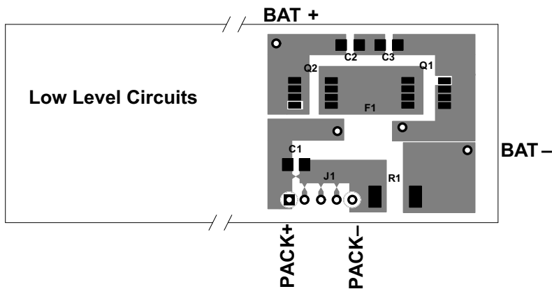
图 8-2. 分离高电流部分和低电流部分可提高抗噪能力
