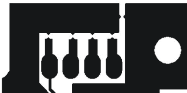
图 8-7. 建议的火花隙模式有助于保护通信线路免受 ESD 影响
