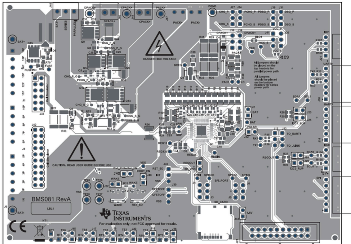
图 8-8. 顶层
