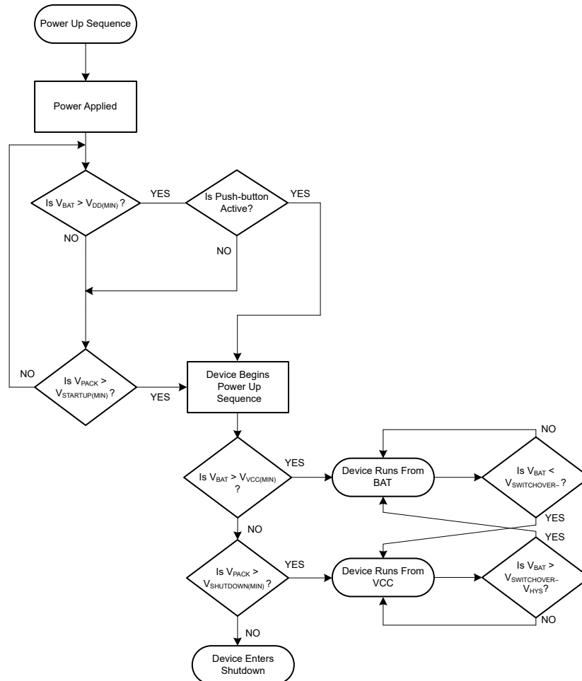
图 7-1. 上电序列
