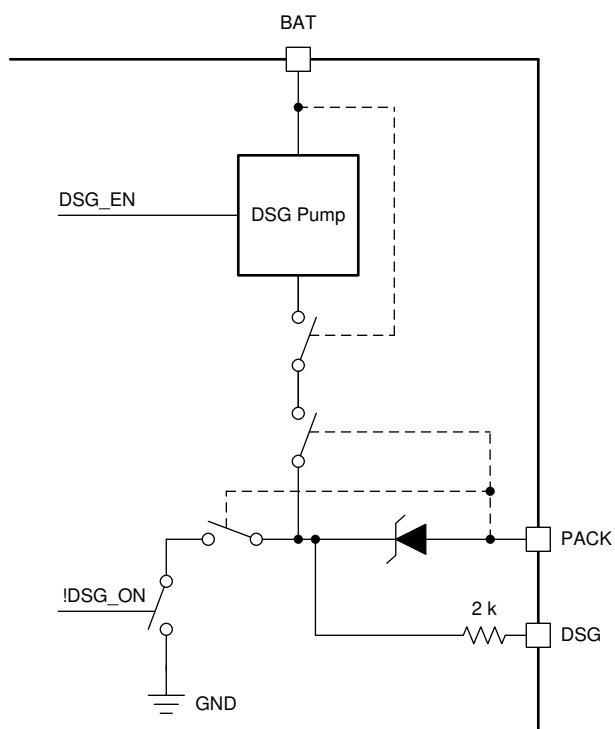
图 5-6. DSG 引脚
