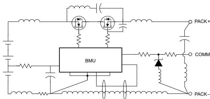
图 8-2. 分离高电流部分和低电流部分可提高抗噪能力
