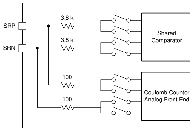
图 5-1. SRx 引脚
