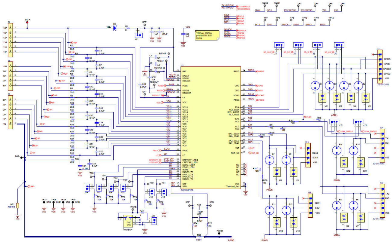
图 8-1. 典型应用
