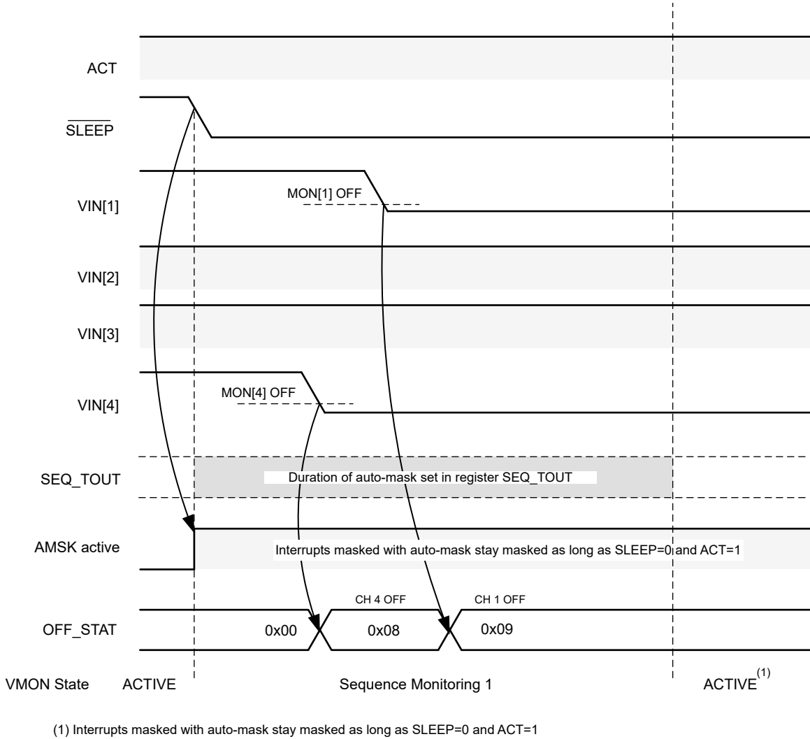
图 7-14. SLEEP 1→0 转换
