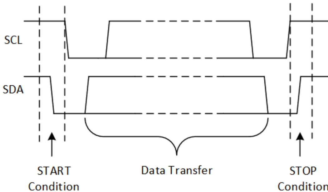
图 7-6. I 2 C START 和 STOP 条件
