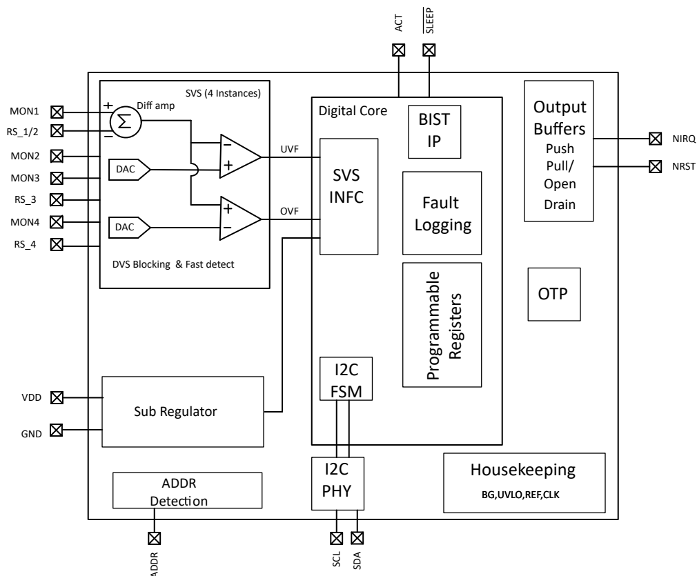
图 7-2. TPS388R04-Q1 方框图
