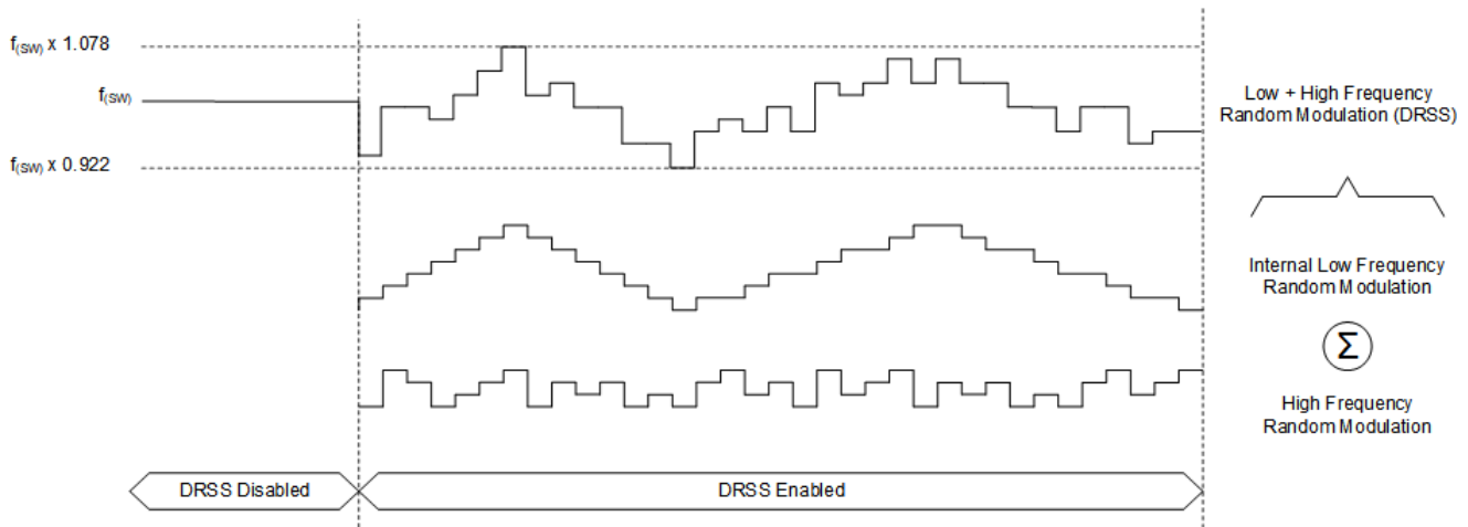
图 6-10. 双随机展频
