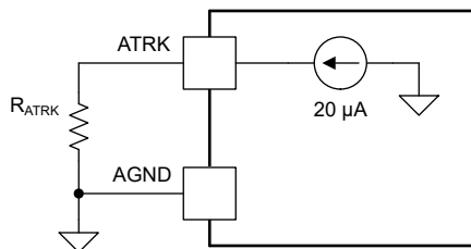
图 6-15. 使用电阻进行 V_{OUT} 编程
