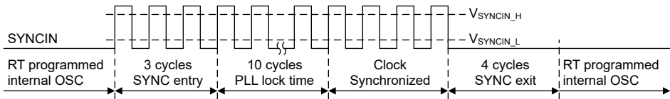
图 6-9. 时钟同步
