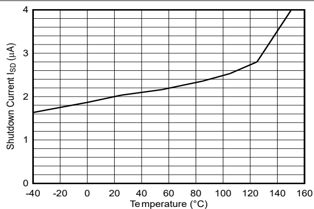
图 5-2. 关断电流与温度间的关系
