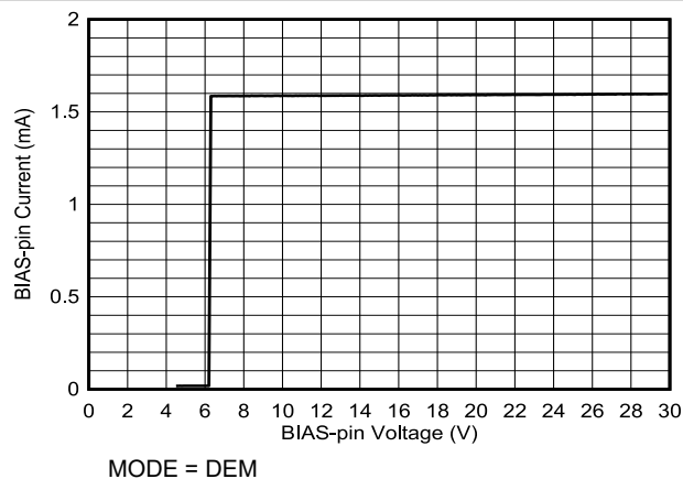
图 5-5. BIAS 引脚静态电流与 BIAS 引脚电压之间的关系
