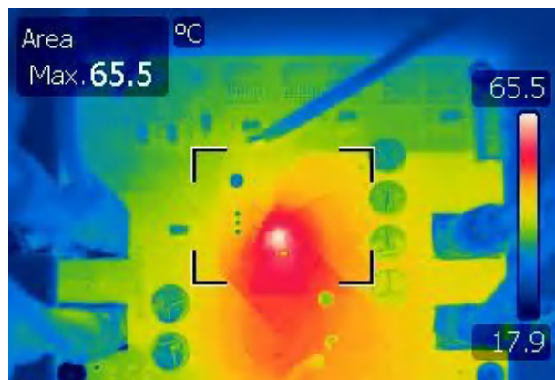
图 7-15. V_{IN} = 14.4V , V_{OUT} = 24V , P_{OUT} = 240W , 自然对流
