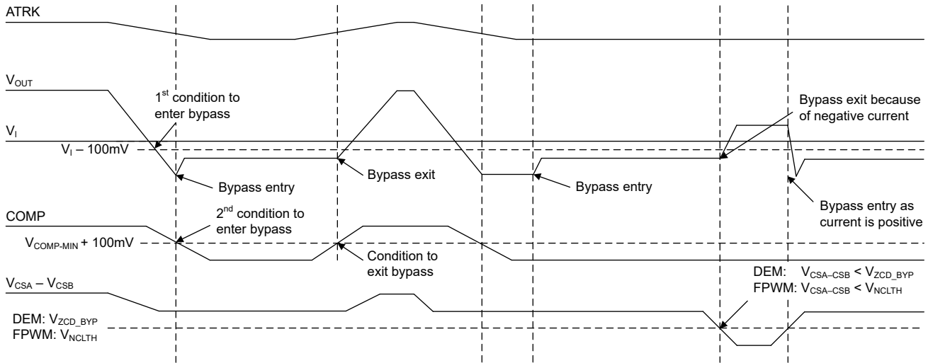
图 6-12. 进入、退出旁路模式
