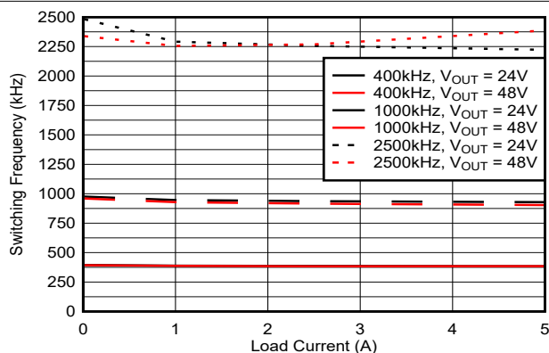
图 5-13. 开关频率与负载电流间的关系
