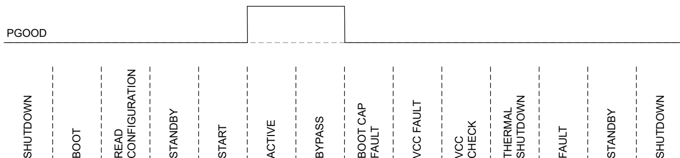
图 6-19. 所有器件状态的 PGOOD 状态
