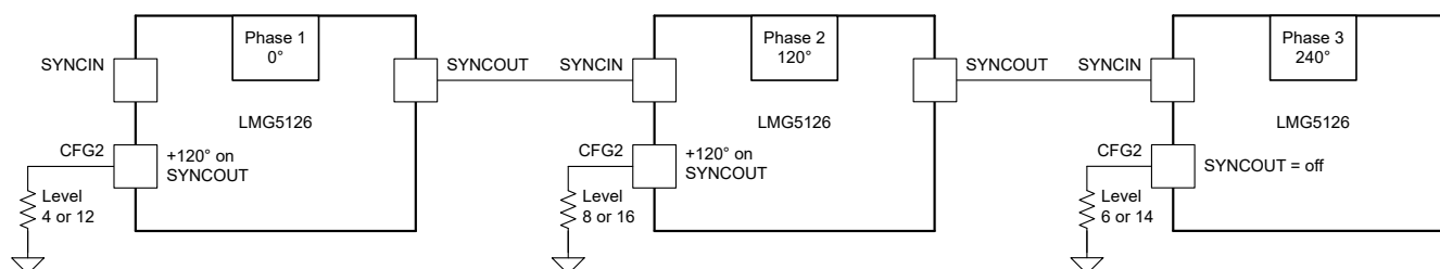
图 6-6. 三器件配置
