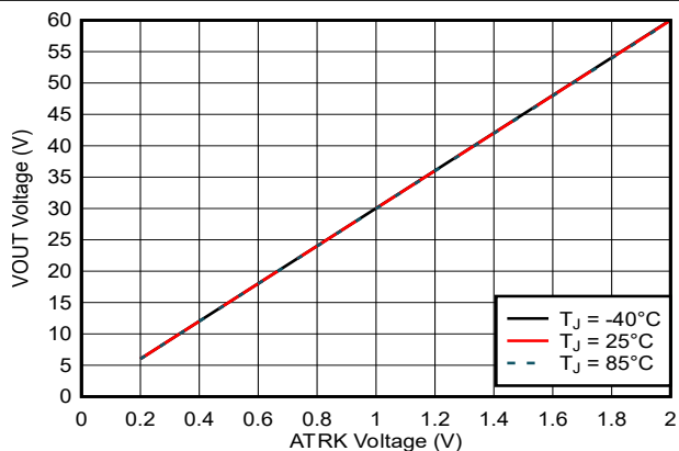
图 5-18. V_{\text{OUT}} 电压与 V_{\text{ATRK}} 电压间的关系
