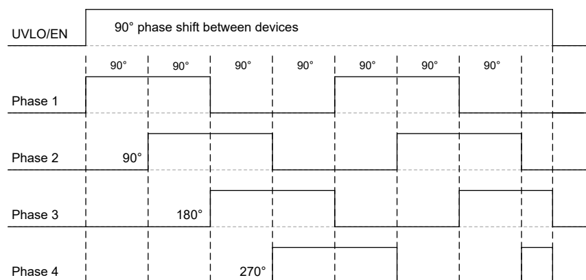
图 6-4. 四器件四相运行
