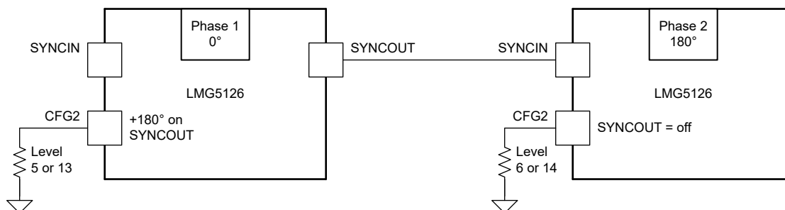
图 6-5. 二器件配置
