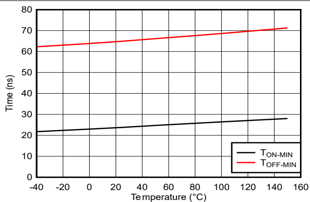
图 5-14. 最短可控导通时间与温度间的关系
