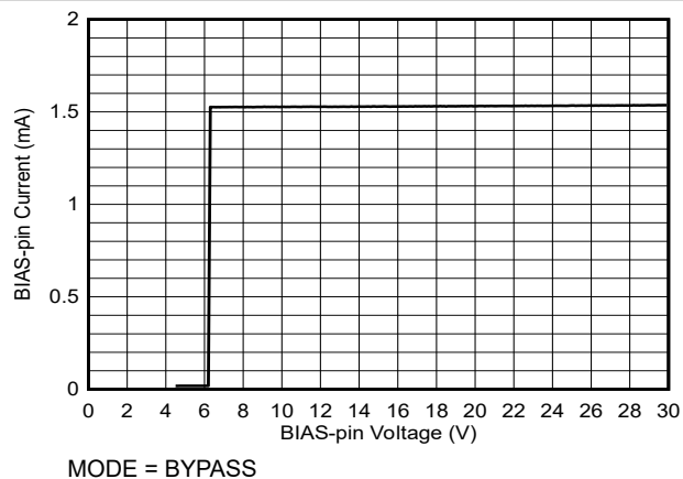
图 5-6. BIAS 引脚静态电流与 BIAS 引脚电压之间的关系
