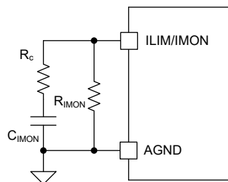
图 7-6. ILIM/IMON 引脚配置
