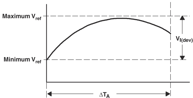
图 7-4. \alpha_{V_{ref}} 平均温度系数
