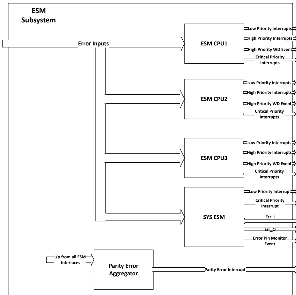
图 7-3. ESM-SS 方框图
