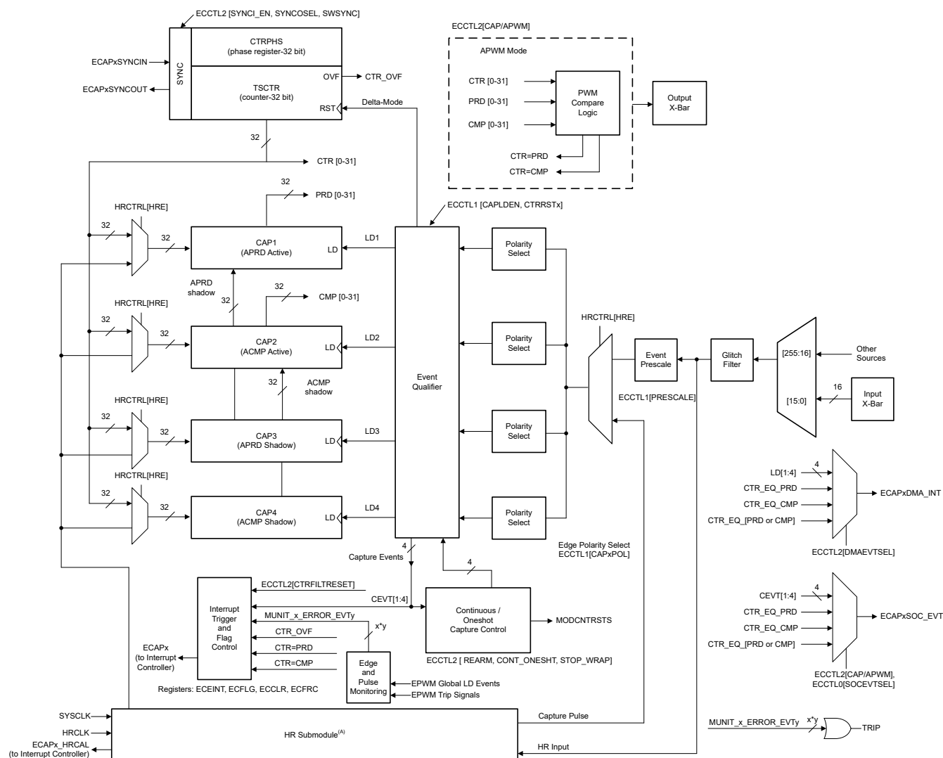
图 6-62. eCAP 方框图
