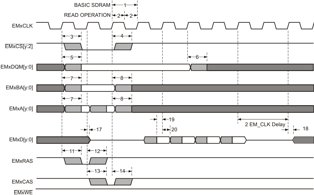
图 6-26. 基本 SDRAM 读取操作
