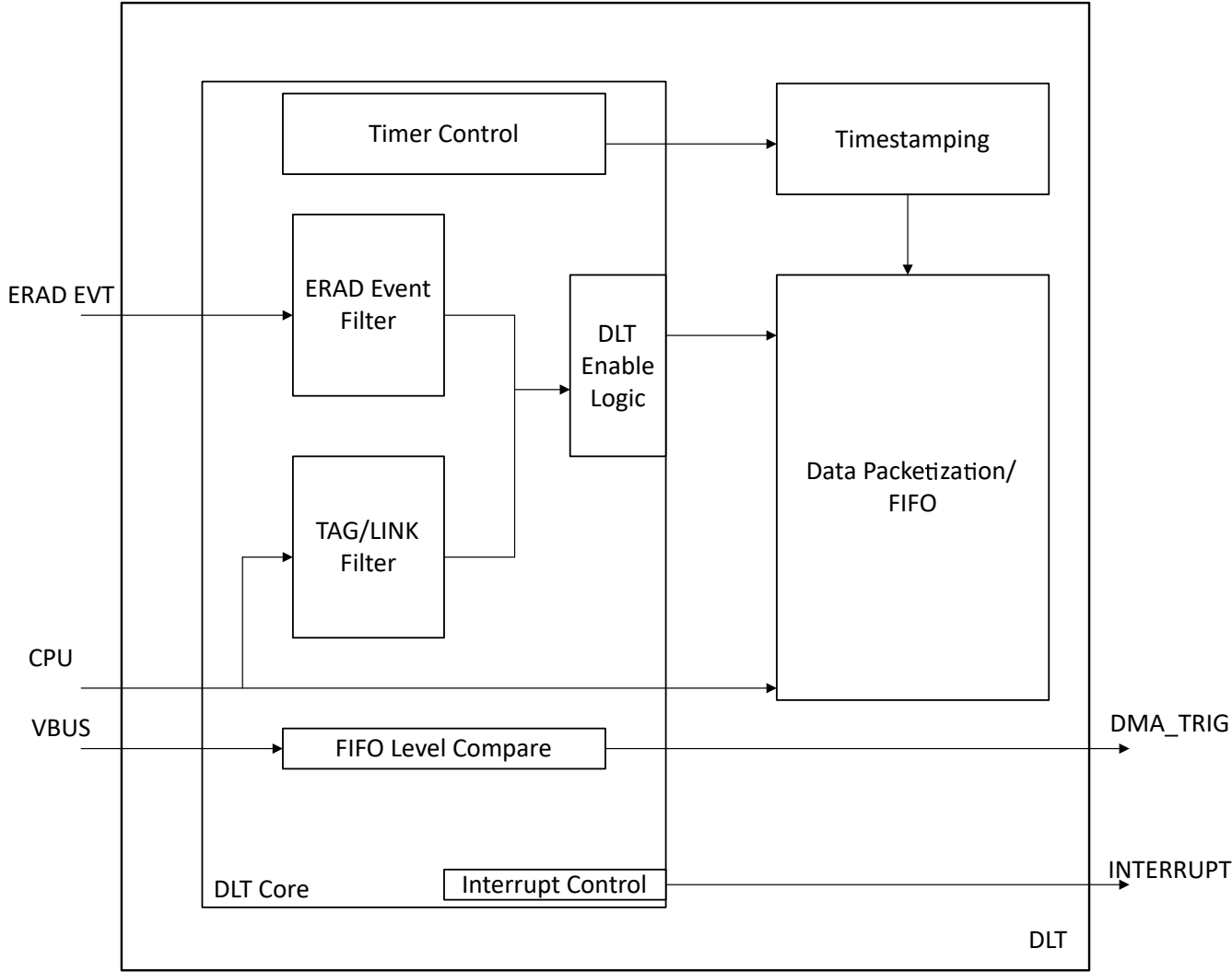
图 7-17. DLT 方框图
