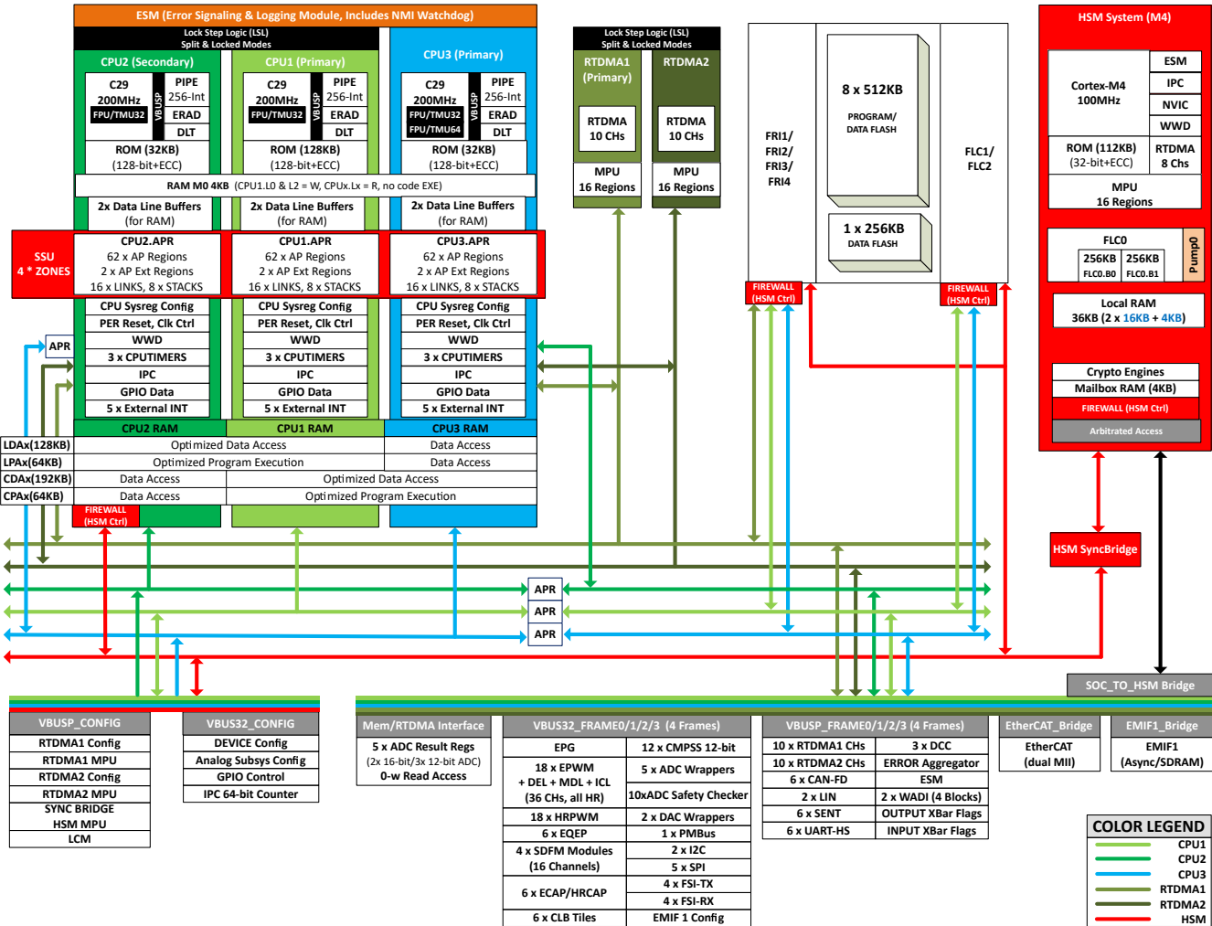
图 3-1. 功能方框图
