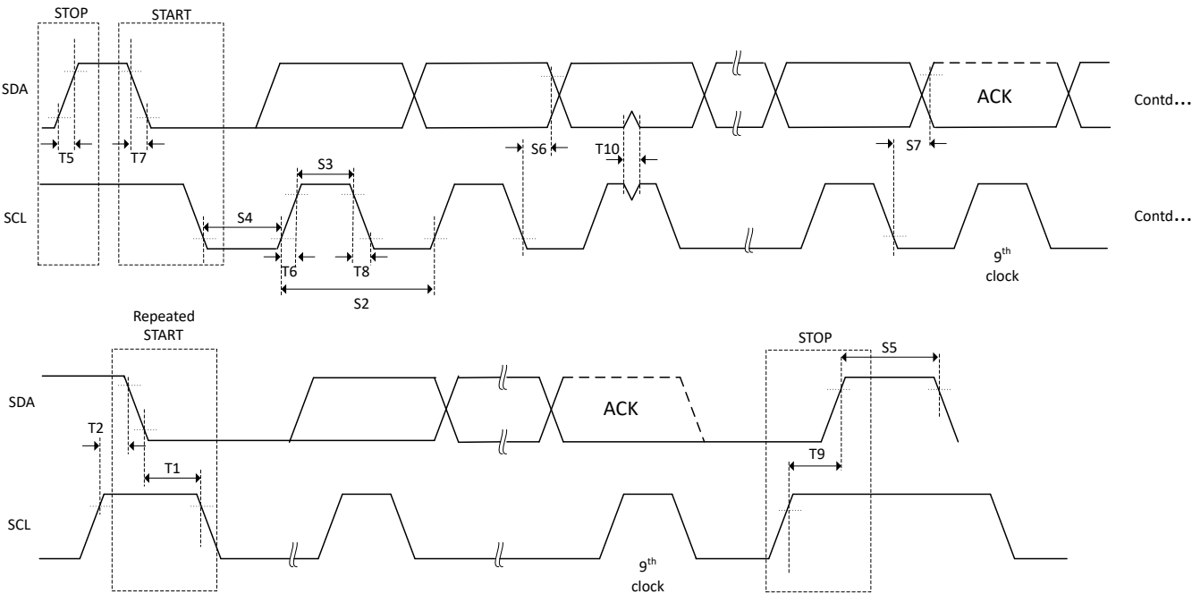
图 6-83. I2C 时序图
