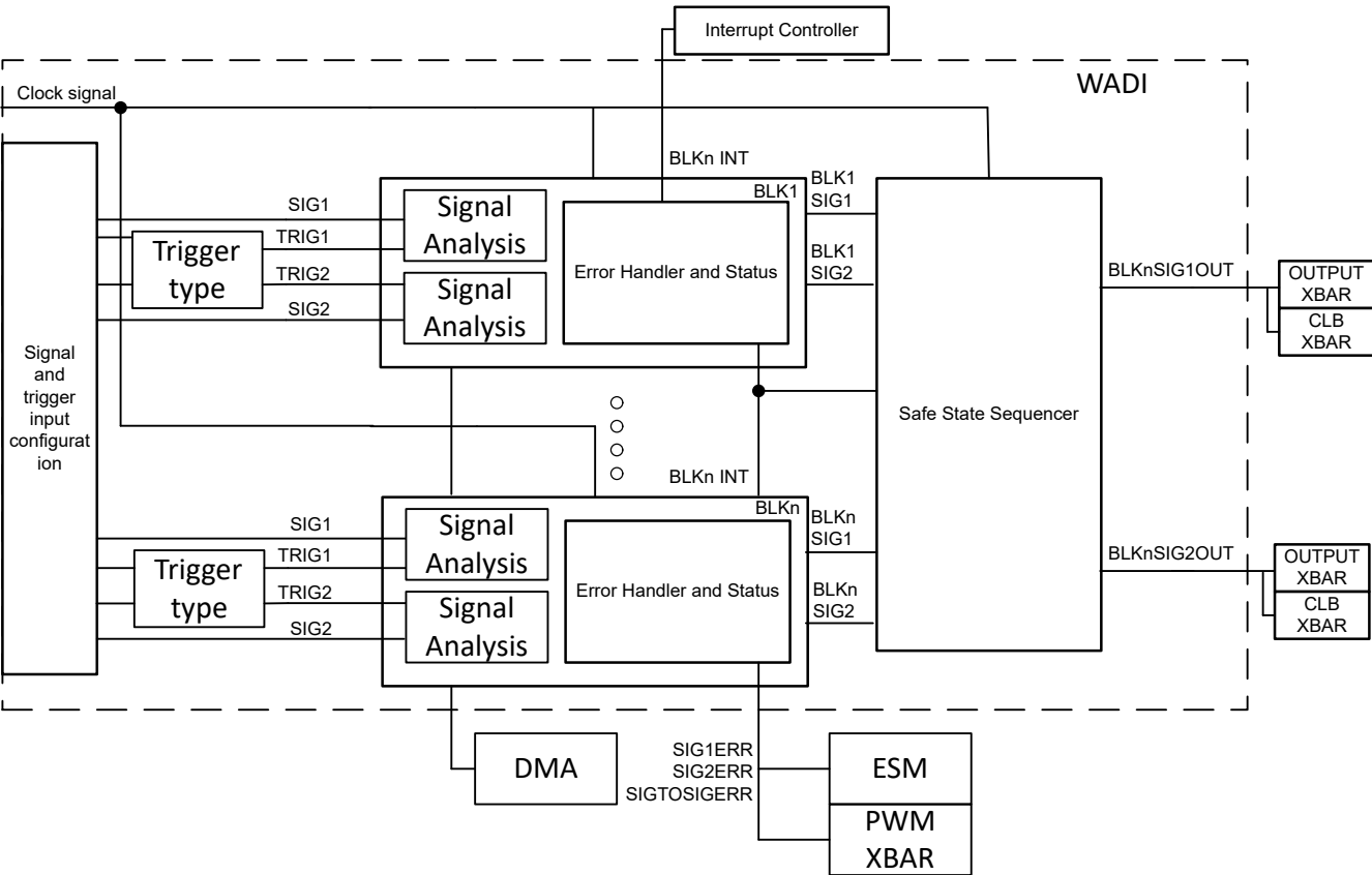
图 7-18. WADI 方框图
