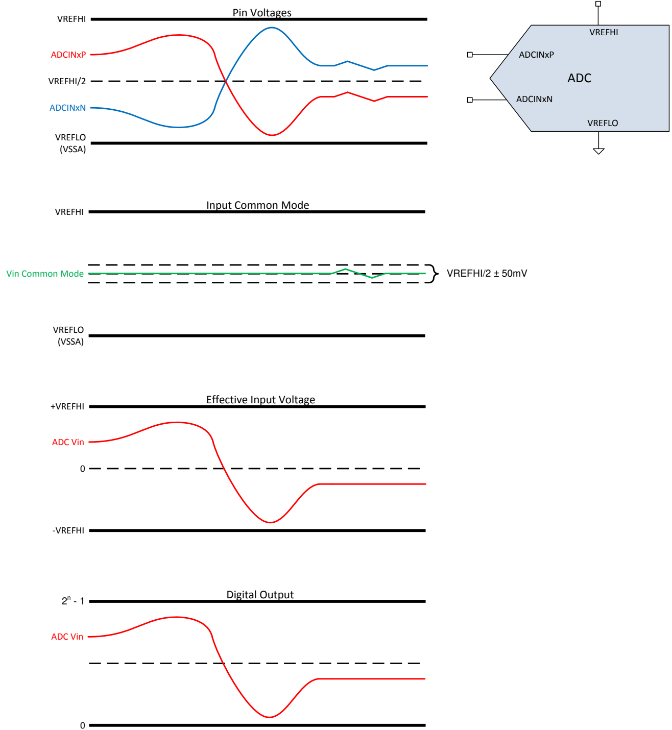
图 6-36. 差分信号模式
