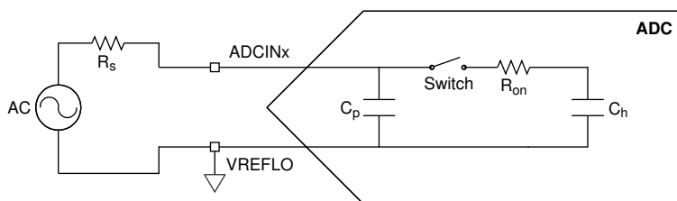
图 6-47. 单端输入模型
