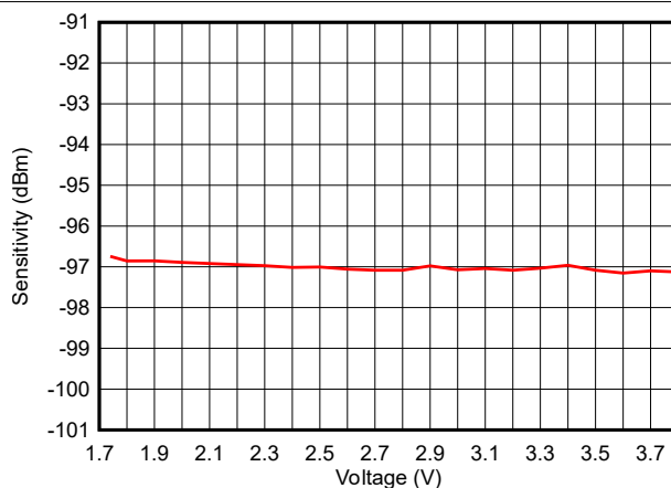
图 7-18. 灵敏度与电源电压 (VDDS) 间的关系 (BLE 1Mbps , 2.44GHz )
