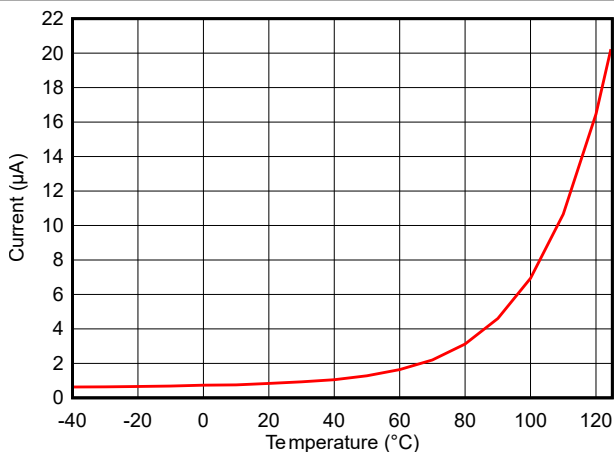
图 7-7. 待机模式 (MCU) 电流与温度间的关系 (SRAM 和部分寄存器保留, 启用 RTC), V_{\text{DDS}} = 3.3\text{V}
