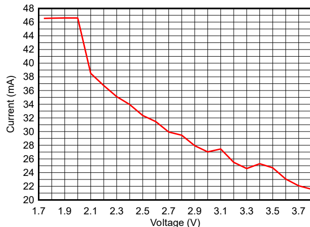
图 7-13. TX 电流与电源电压 (VDDS) 间的关系 ( BLE 1Mbps , 2.44GHz , +10dBm )
