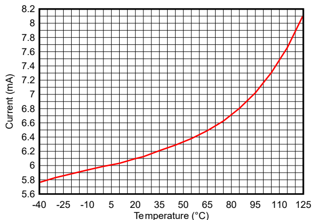
图 7-8. RX 电流与温度间的关系 (BLE 1Mbps, 2.44GHz), V_{\text{DDS}} = 3.3\text{V}
