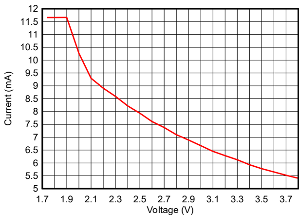
图 7-9. RX 电流与电源电压 ( V_{\text{DDS}} ) 间的关系 (BLE 1Mbps, 2.44GHz)
