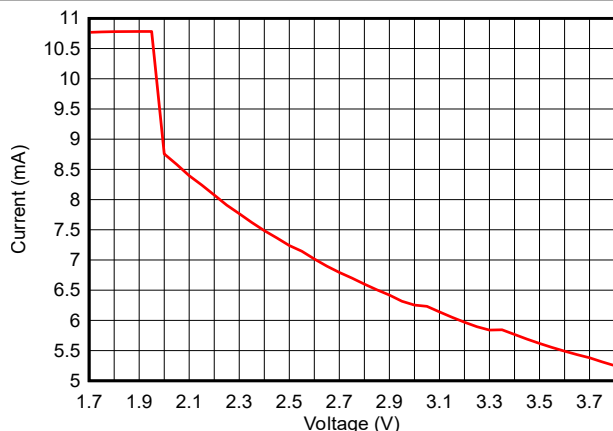
图 7-6. 工作模式 (MCU) 电流与电源电压 ( V_{\text{DDS}} ) 间的关系 (运行 CoreMark)
