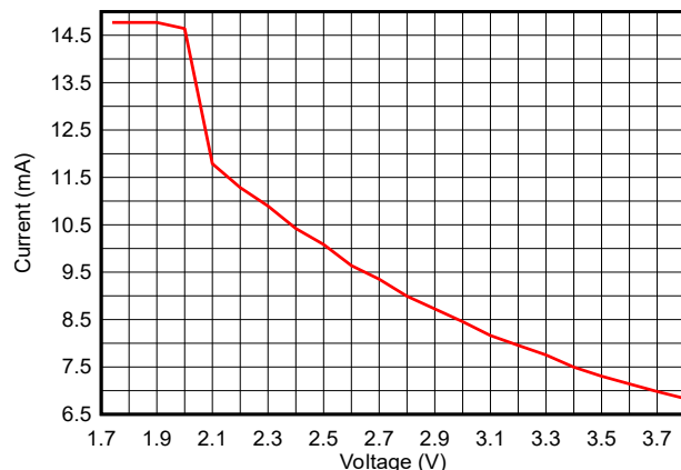
图 7-12. TX 电流与电源电压 (VDDS) 间的关系 ( BLE 1Mbps , 2.44GHz , 0dBm )
