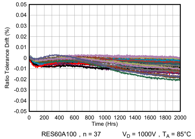
图 5-4. 长期漂移
