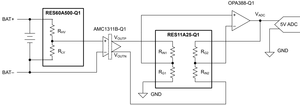
图 7-6. 采用 RES60A-Q1 和 AMC1311B-Q1 的直流总线测量
