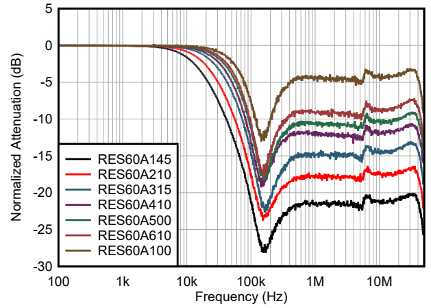
图 5-2. 衰减与频率间的关系，已补偿
