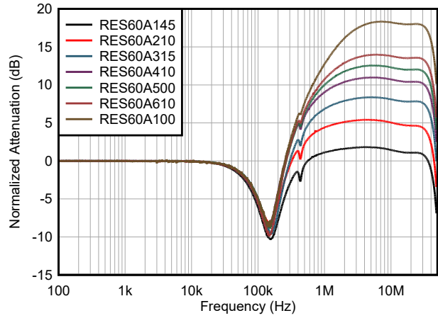
图 5-1. 衰减与频率间的关系，未补偿
