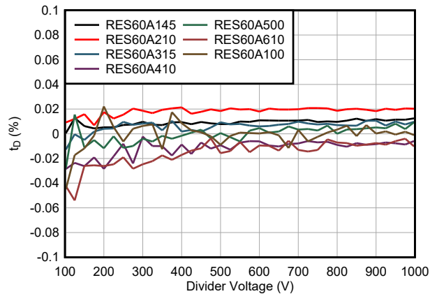
图 5-3. t_D 与分压器电压间的关系
