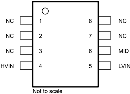
图 4-1. DWV 封装，8 引脚 SOIC（顶视图）
