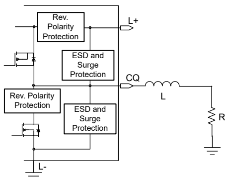
图 9-3. P 开关模式
