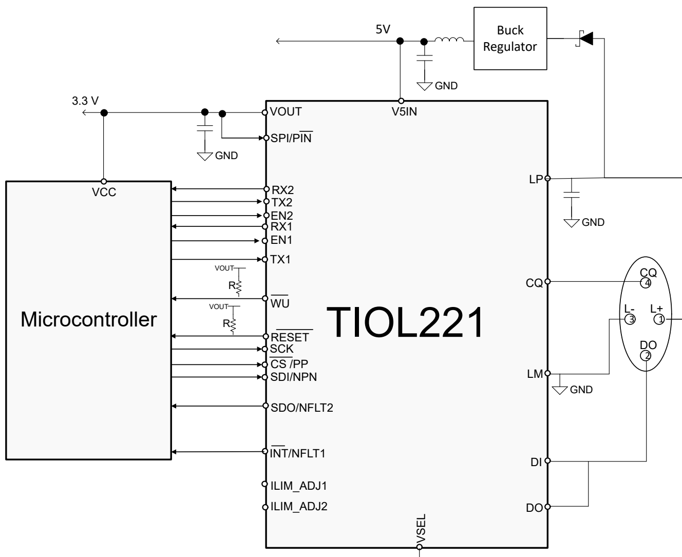
图 9-1. 典型应用原理图 ( SPI 模式 )
