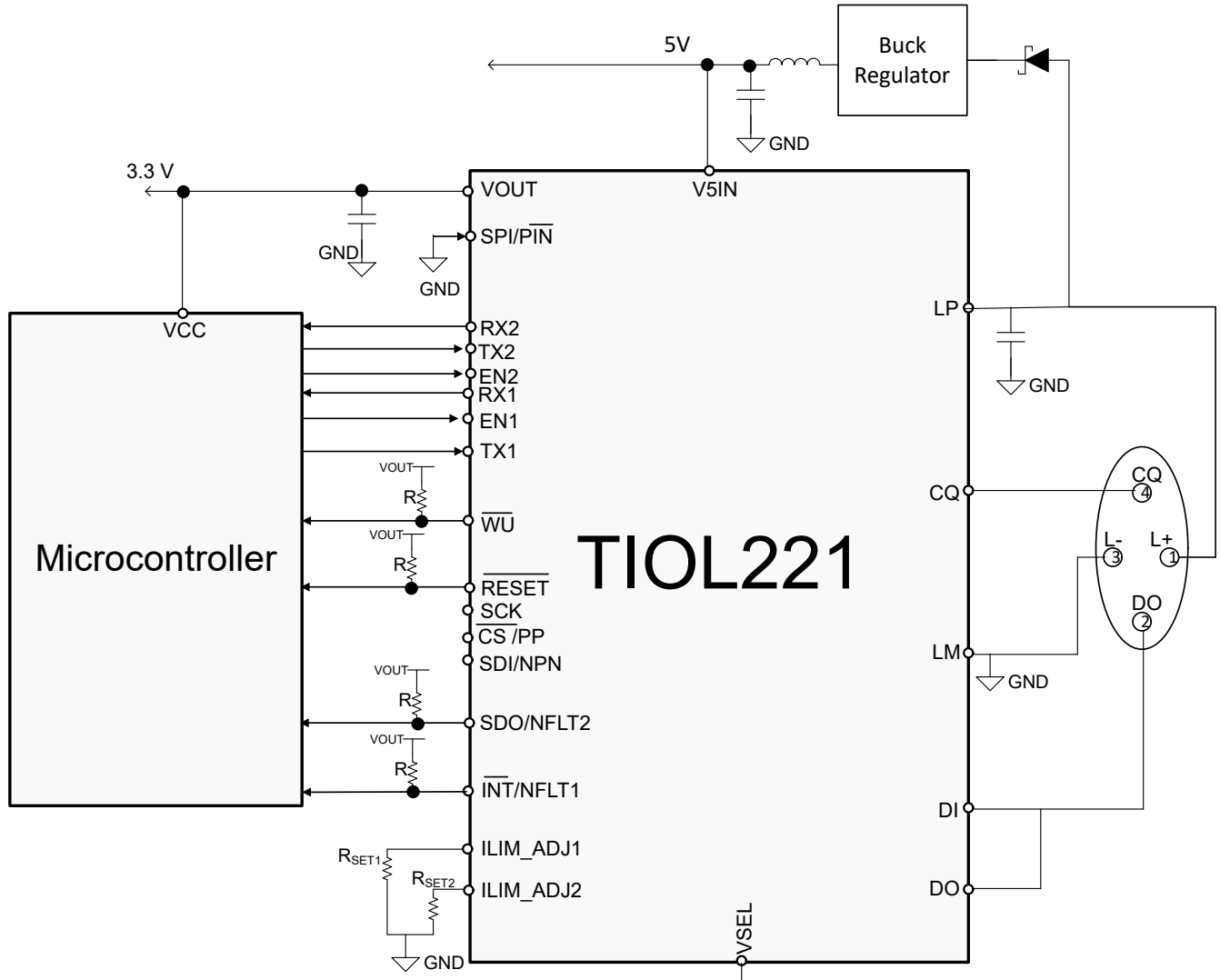
图 9-2. TIOL221 应用原理图 ( 引脚模式 )
