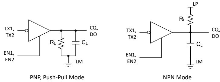
图 6-1. 驱动器开关的测试电路
