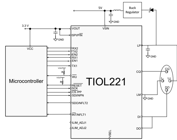
典型应用图
