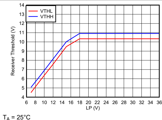
图 5-5. CQ、DI 接收器阈值边界
