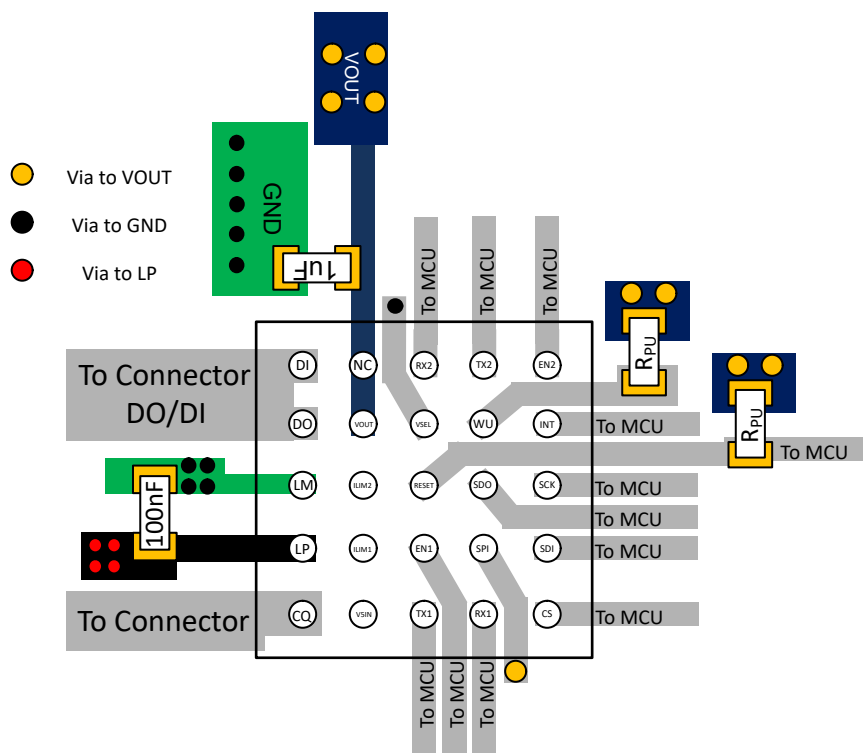
图 9-9. DSBGA 布局示例 (显示的是 SPI 模式)
