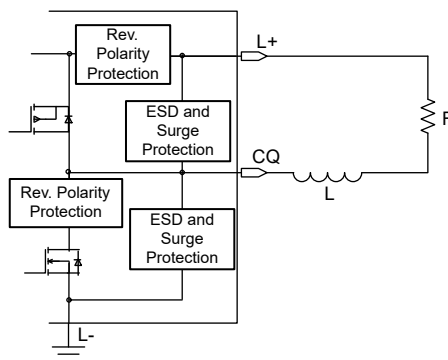
图 9-4. N 开关模式
