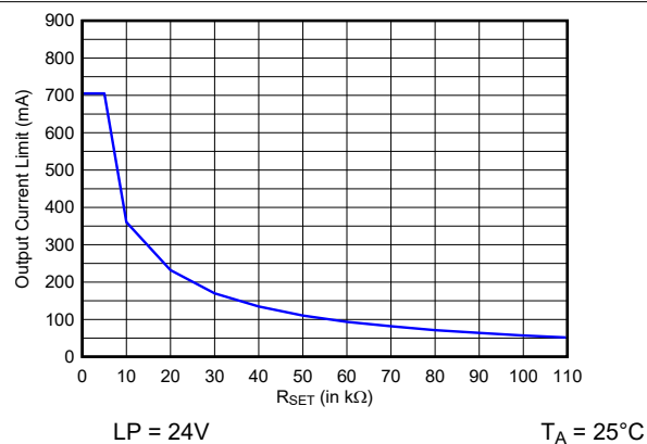
图 5-4. CQ、DO 电流限值与 0-5k \Omega 范围内的 R SETx 1
