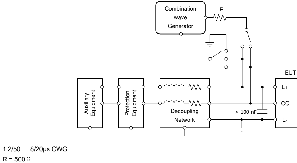
图 7-4. 浪涌测试设置
