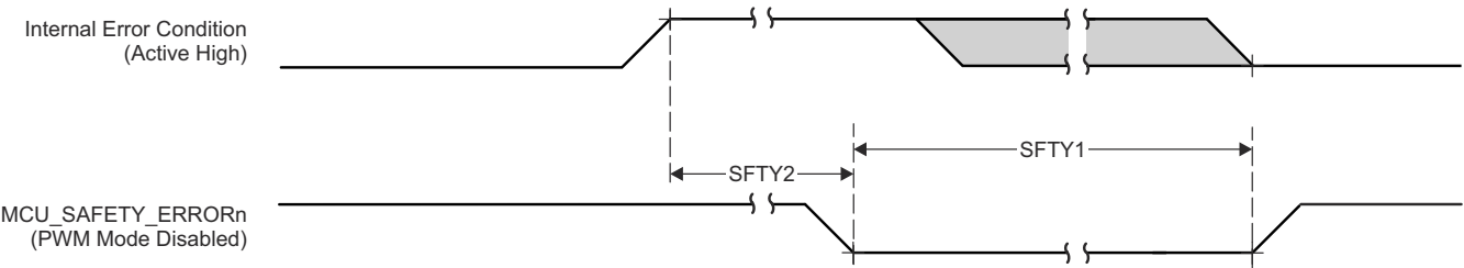
图 6-21. MCU_SAFETY_ERRORn 开关特性
