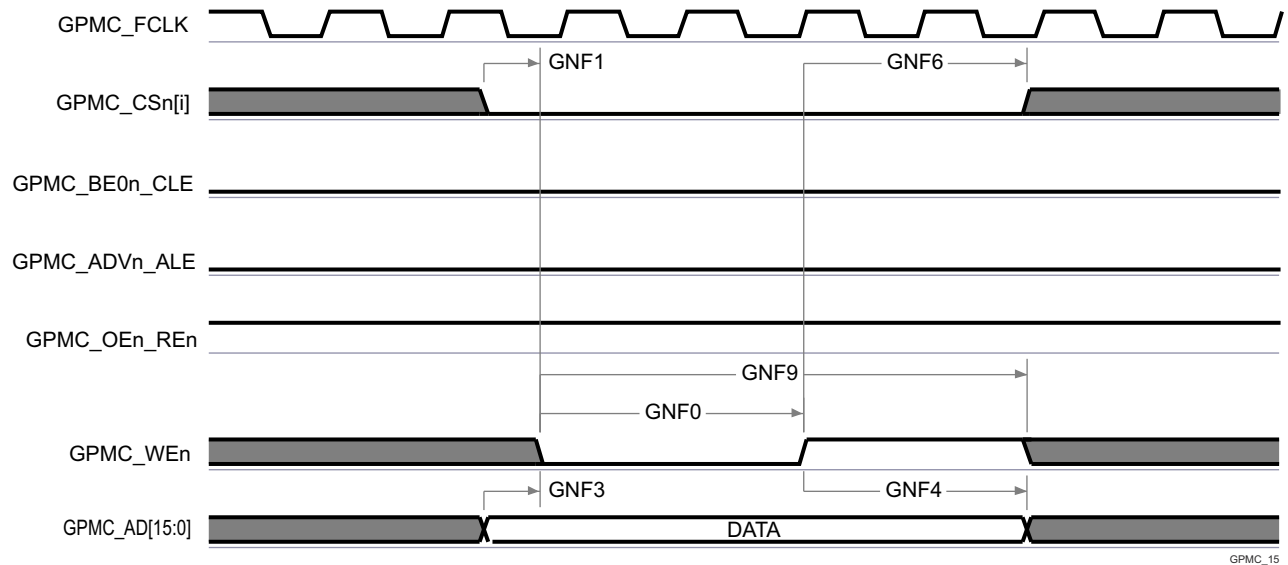
图 6-66. GPMC 和 NAND 闪存 - 数据读取周期
