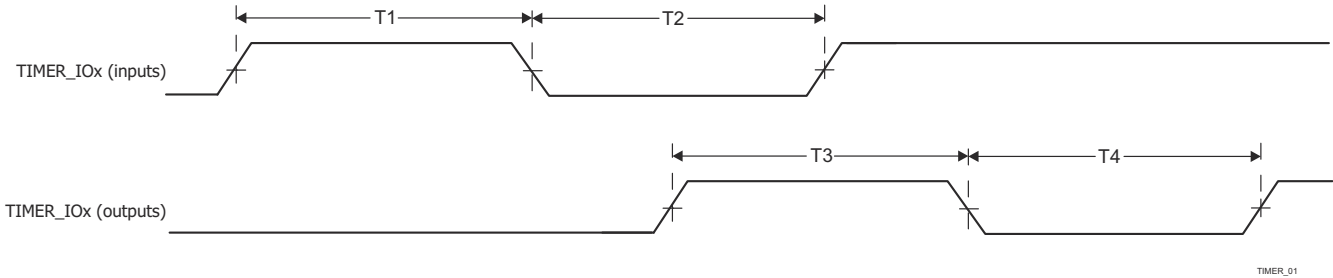
图 6-117. 计时器时序
