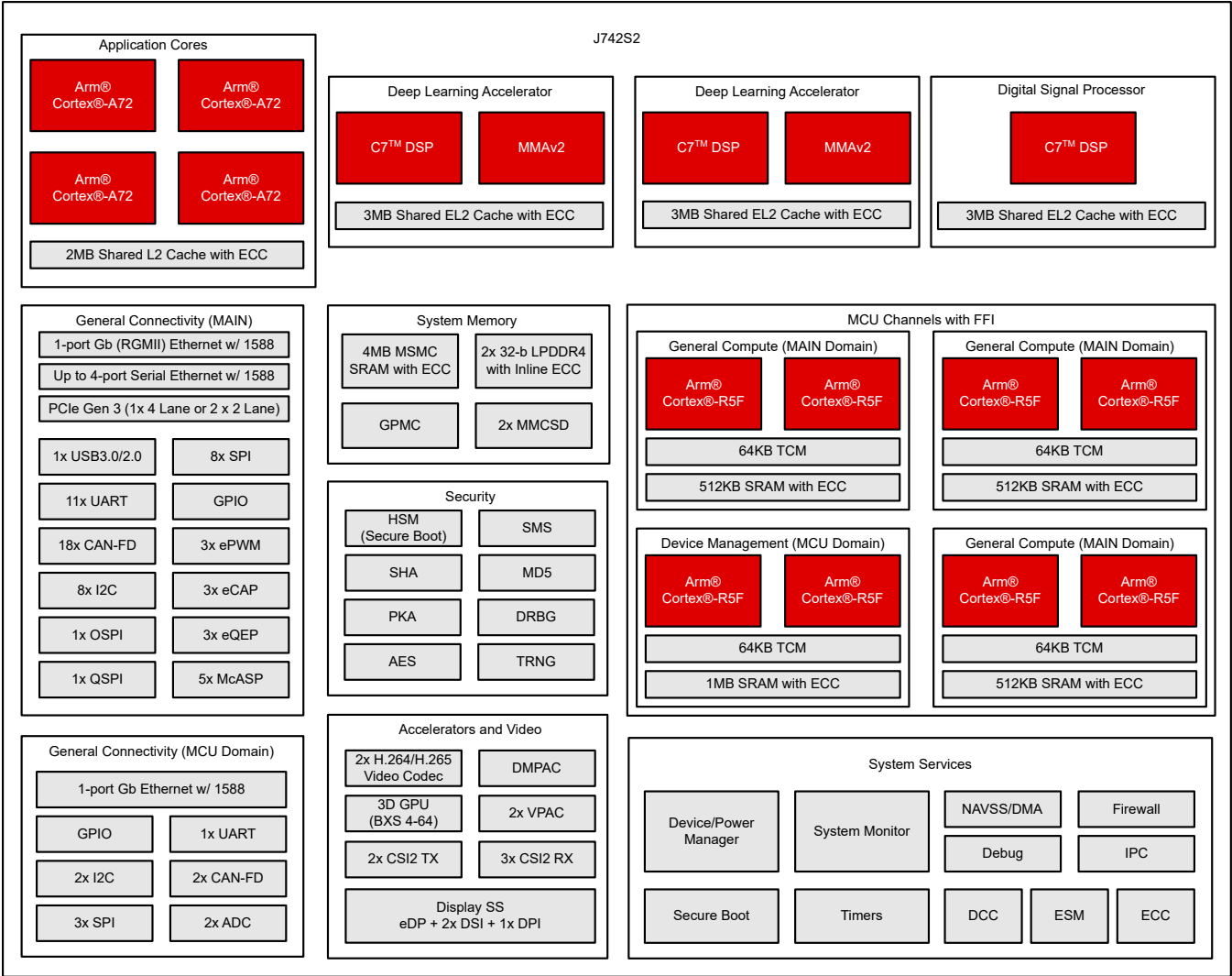
图 3-1. 功能方框图
