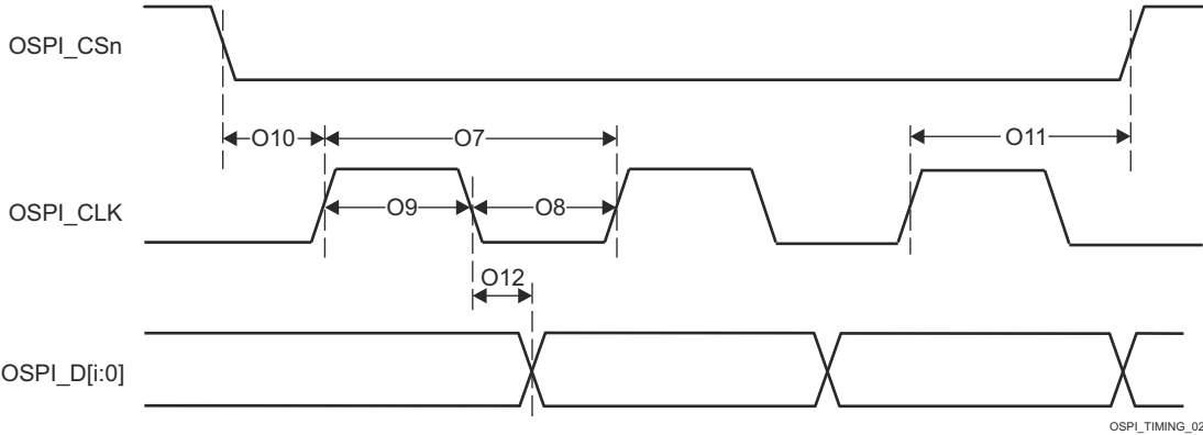
图 6-111. OSPI0/1 开关特性 - Tap SDR , 无环回
