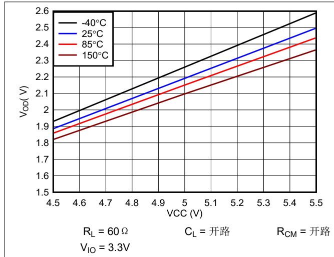
图 5-1. V_{OD(DOM)} 与 V_{CC} 和温度间的关系
