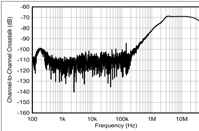
图 5-19. 通道间串扰
