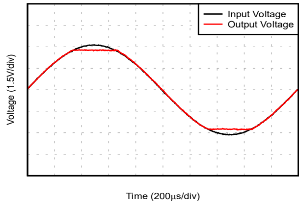
图 5-20. 无相位反转
