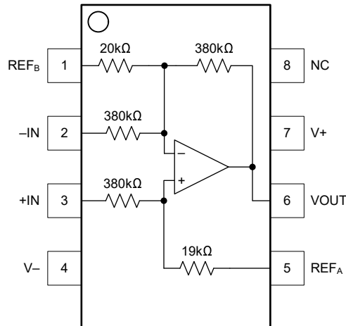
INA117 D 封装 (顶视图)
