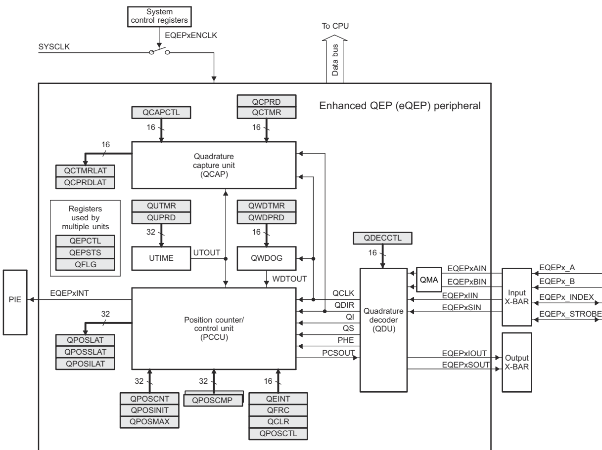
图 6-63. eQEP 方框图
