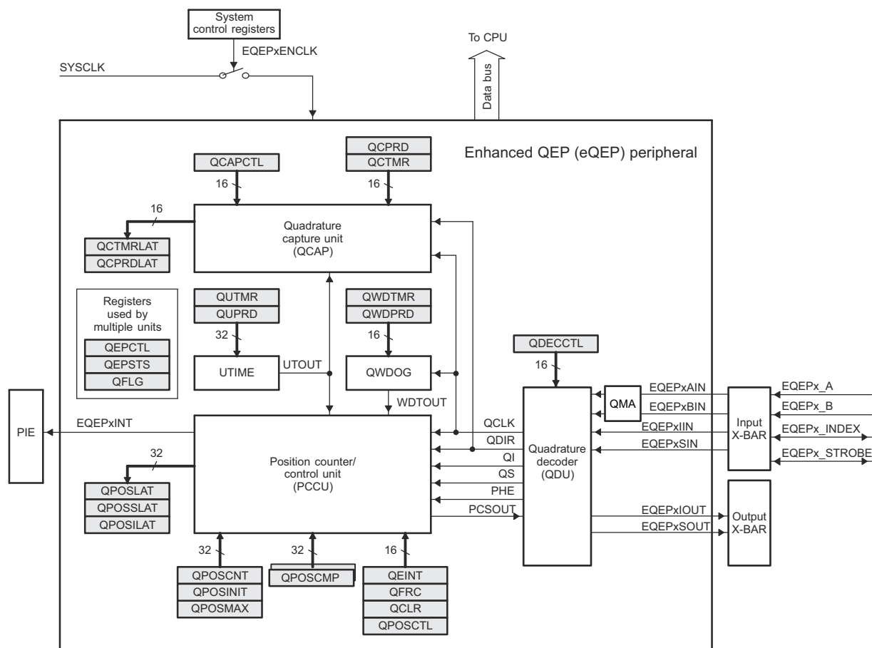
图 6-63. eQEP 方框图
