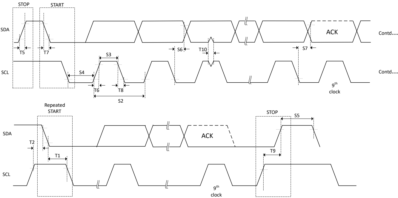
图 6-66. I2C 时序图
