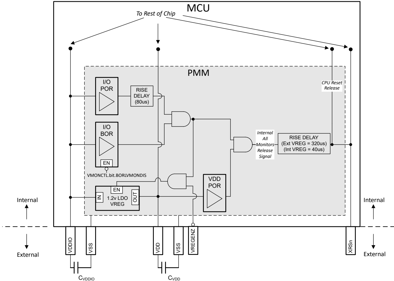
图 6-2. PMM 方框图
