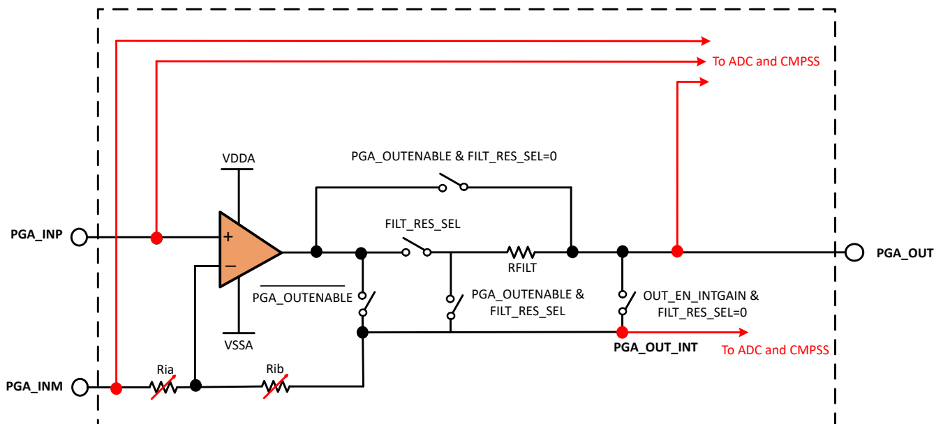
图 6-55. PGA 方框图
