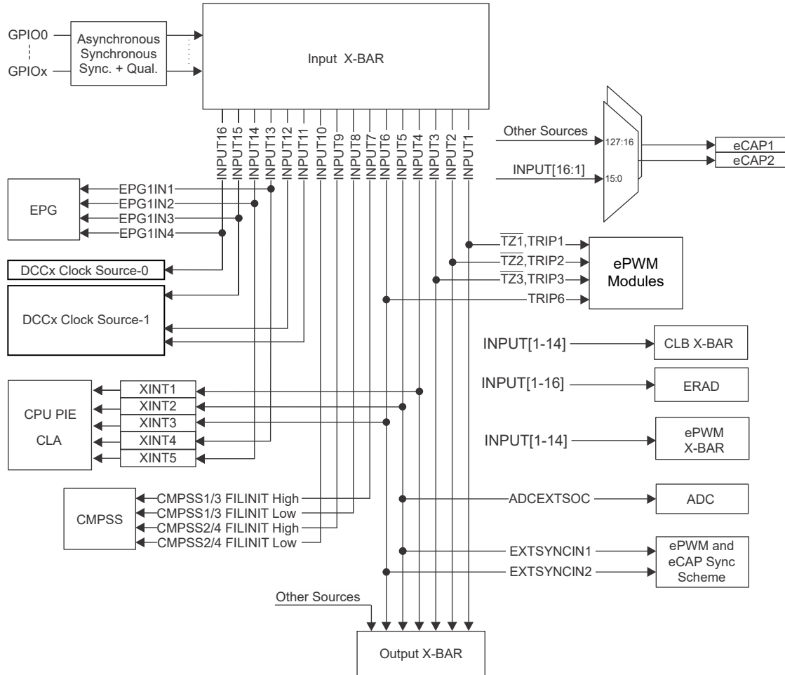
图 5-7. 输入 X-BAR
