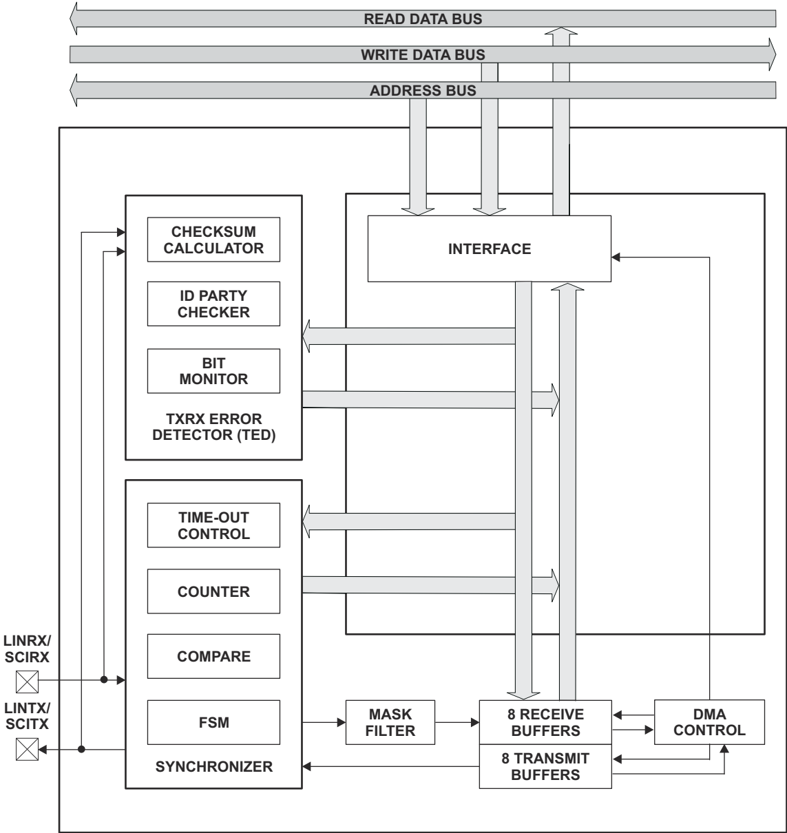
图 6-74. LIN 方框图
