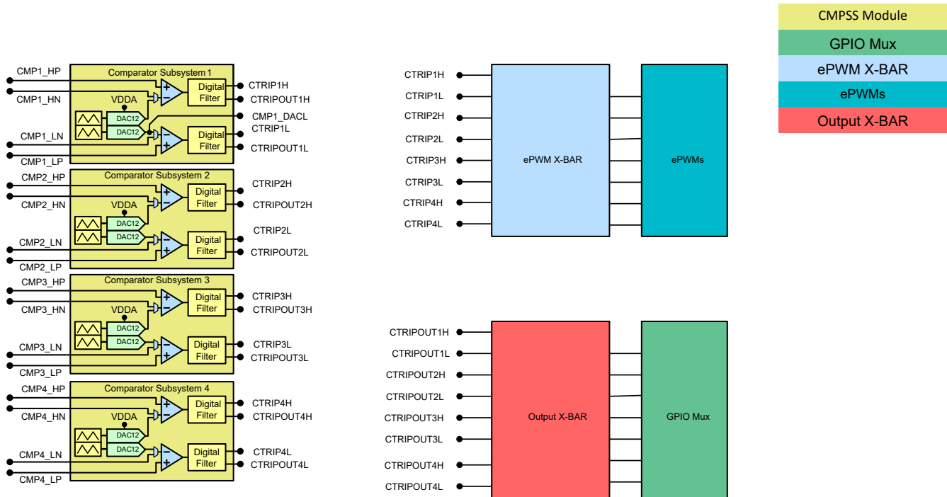
图 6-46. CMPSS 连接
