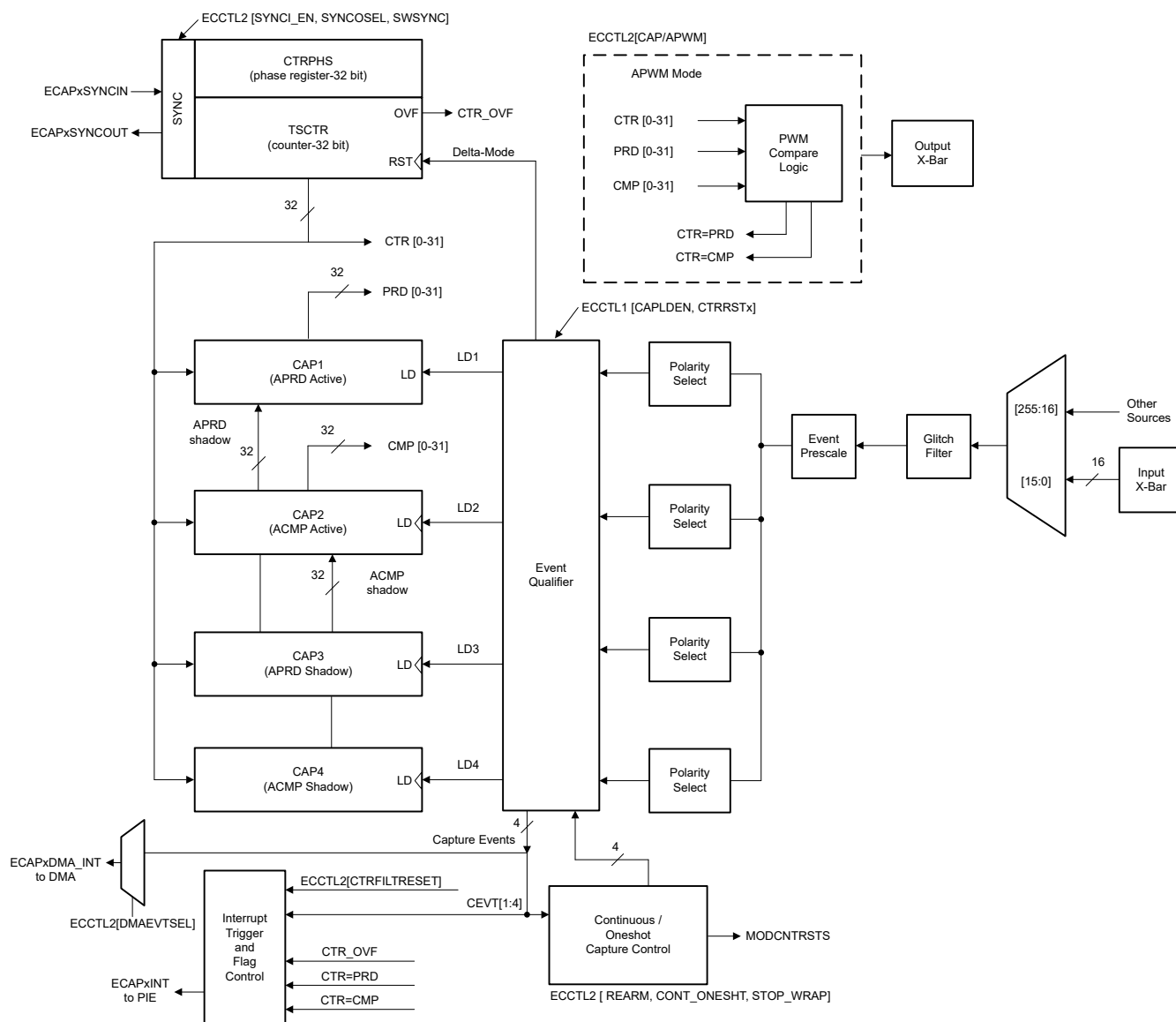
图 6-61. eCAP 方框图
