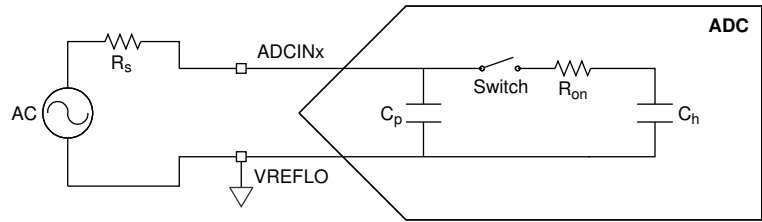
图 6-43. 输入模型
