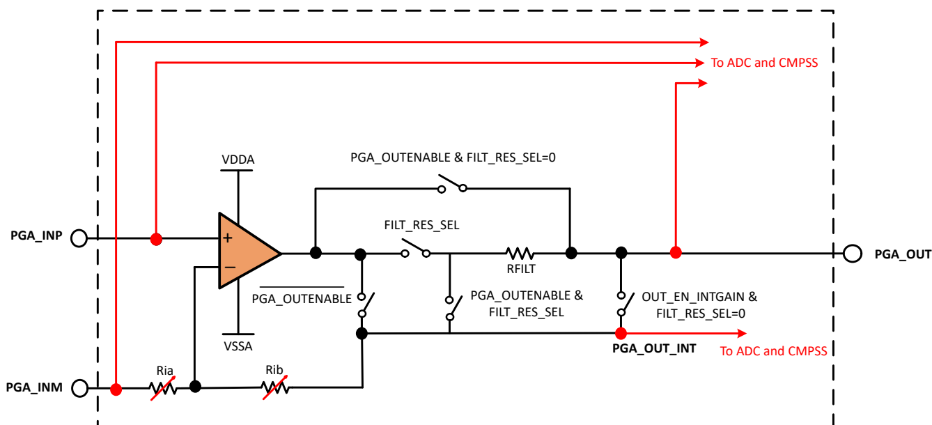
图 6-55. PGA 方框图
