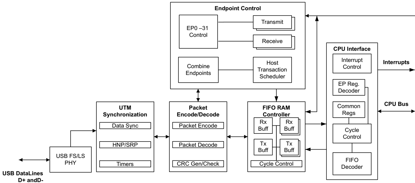
图 6-82. USB 方框图
