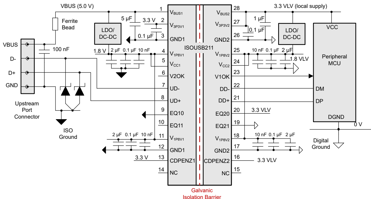
图 8-7. 搭配外部稳压器提供的 1.8V 电源使用 ISOUSB211-Q1
