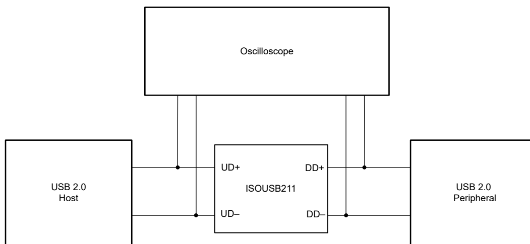
图 6-2. LS、FS 的上行和下行数据包参数和眼图测量
