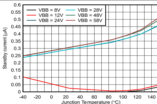
图 6-2. 待机电流
