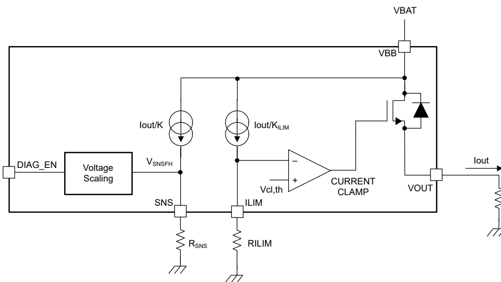
图 7-3. 电流检测和电流限制方框图
