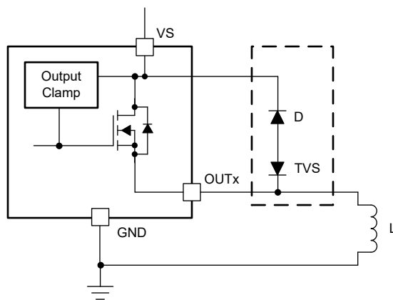
图 7-10. 通过外部电路提供保护
