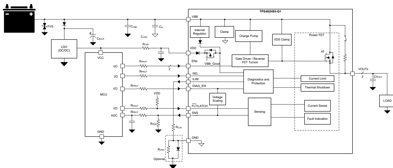
图 8-1. GPIO 版本的典型应用示意图
