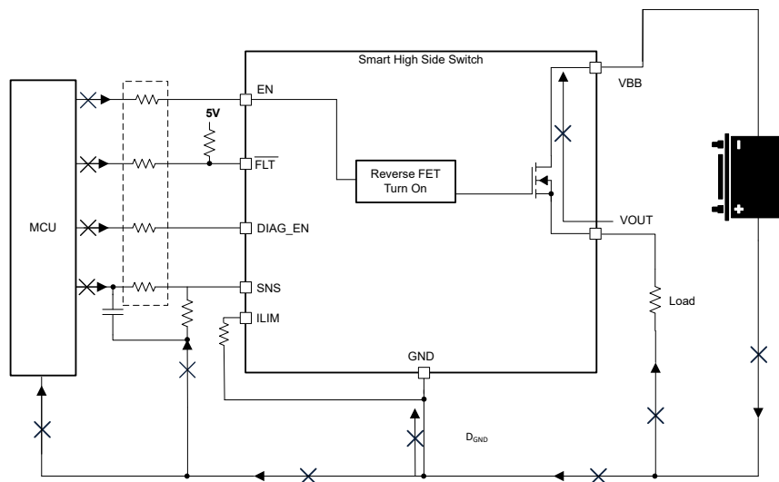
图 7-20. 采用阻断二极管实现反向保护
