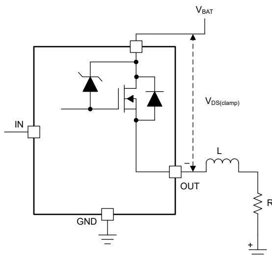
图 7-8. 漏源钳位结构
