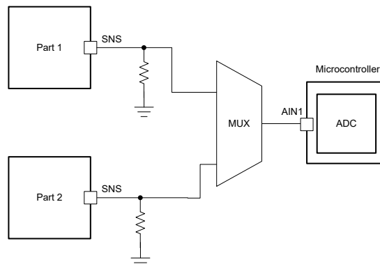
图 7-13. 跨多个器件共享 SNS 方法 2
