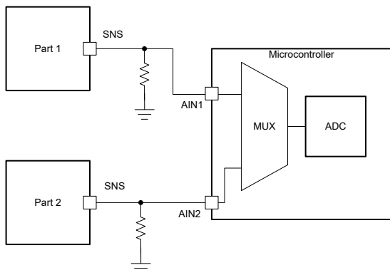
图 7-12. 跨多个器件共享 SNS 方法 1
