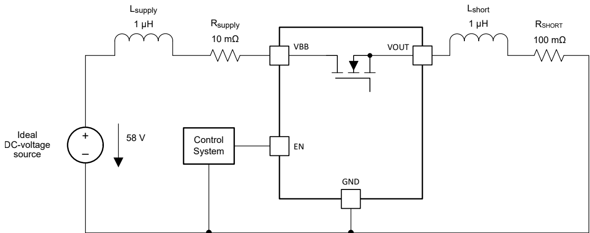
图 7-7. 等效测试电路
