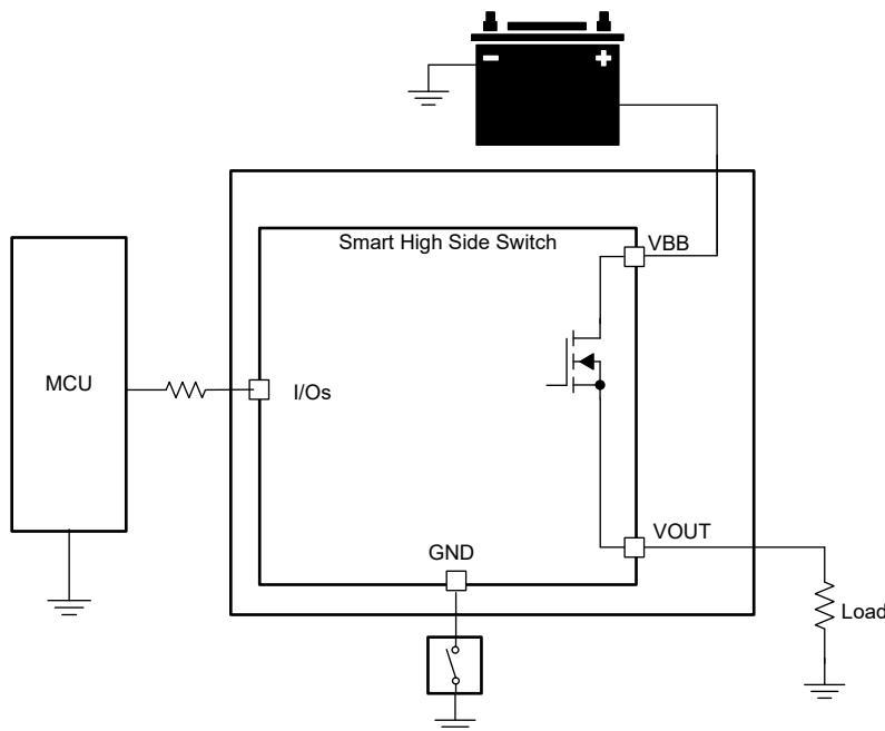
图 7-17. 器件接地失效
