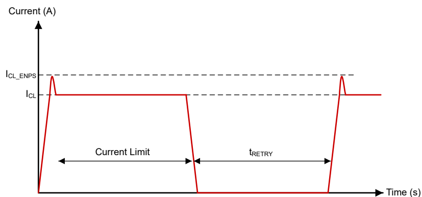
图 7-4. 启用至短路电流限制（自动重试）
