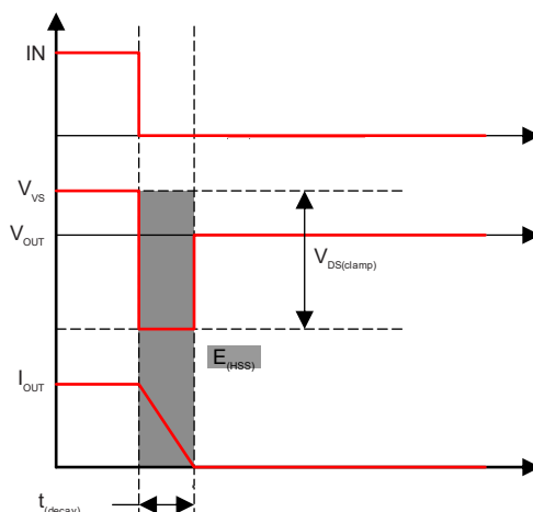
图 7-9. 电感负载关断图
