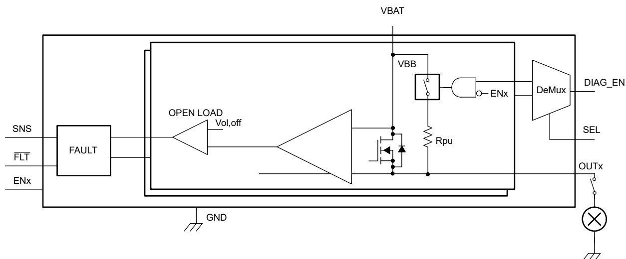
图 7-14. 关断状态下提供开路负载检测
