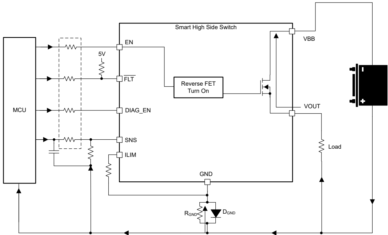
图 7-22. MCU I/O 保护
