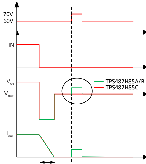
图 7-11. A、B 和 C 版本在电感负载关断工况下的差异
