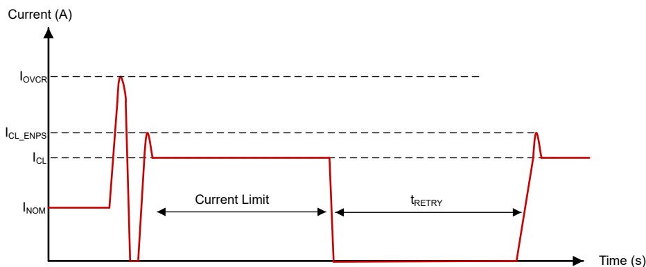
图 7-6. 热短路事件 (自动重试)
