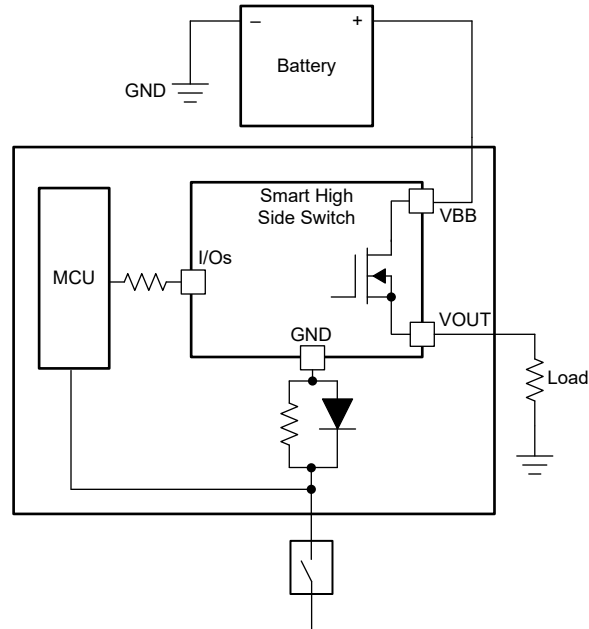
图 7-18. 模块接地失效
