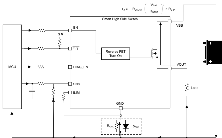
图 7-21. 通过接地网络实现反向保护
