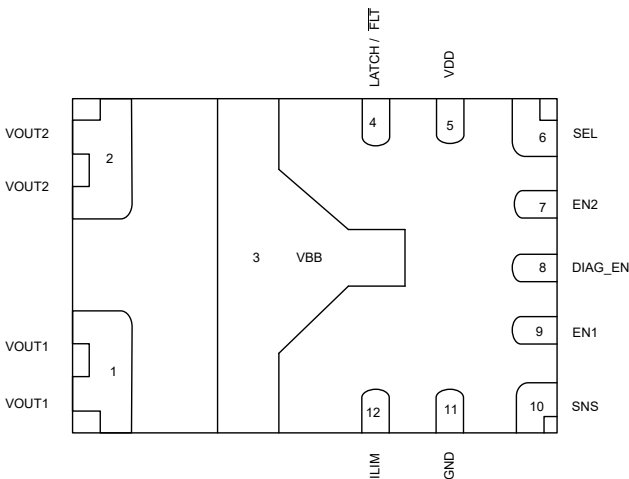
图 5-1. CHU 封装 12 引脚 VQFN-HR 底视图
