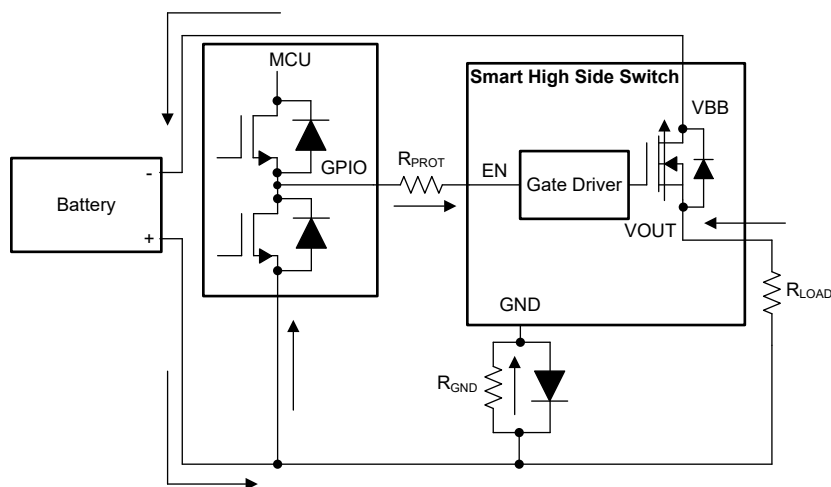
图 7-15. 电池反向电路
