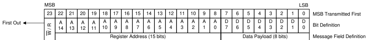
图 8-39. SPI 消息格式
