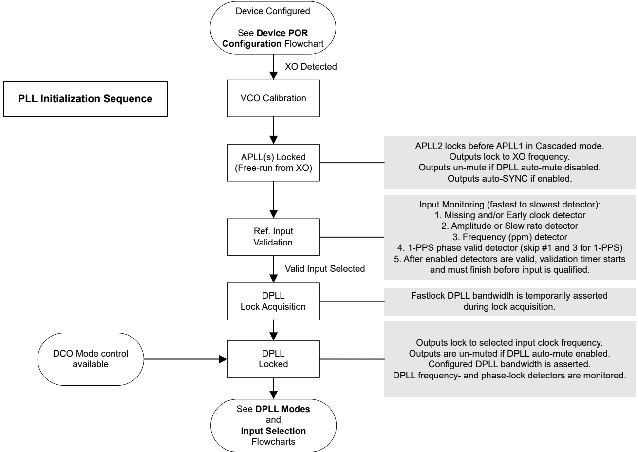
图 8-33. PLL 启动序列
