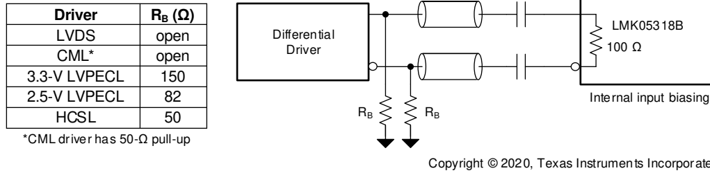
图 8-14. 差分交流耦合至基准 (PRIREF/SECREf) 或 XO 输入
