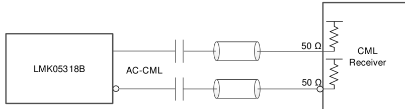
图 8-27. AC-LVDS 输出至带内部端接/偏置的 LVDS 接收器
