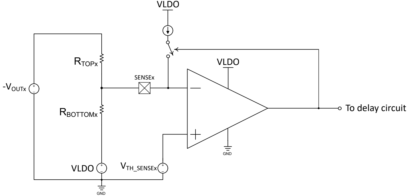
图 9-4. 使用 VLDO 对 TPS7H3xx4 进行负电压监控
