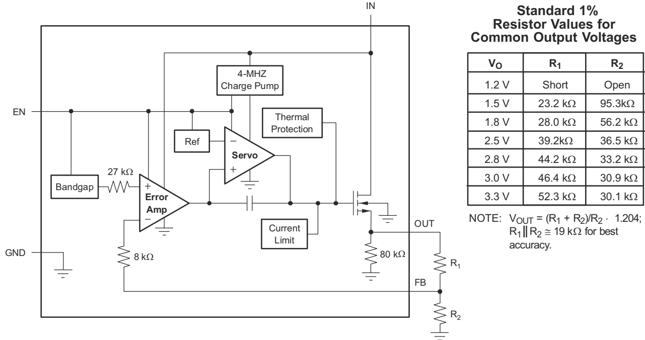
图 6-2. 可调电压版本
