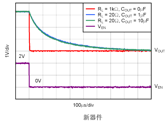
图 5-42. TPS73133 关断响应
