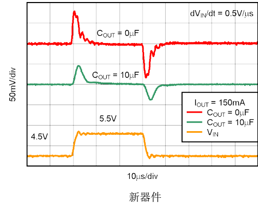
图 5-38. TPS73133 线路瞬态响应
