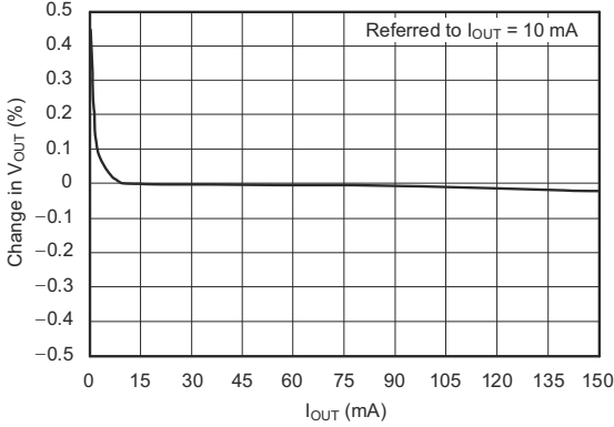
图 5-1. 负载调整率
