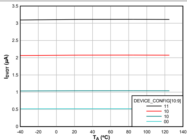
图 6-15. 整个温度范围内的 DVDVT 引脚充电电流
