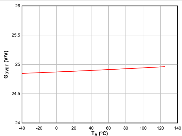
图 6-16. 整个温度范围内的 DVDVT 增益
