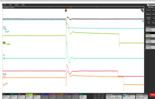
图 6-26. 过流保护
