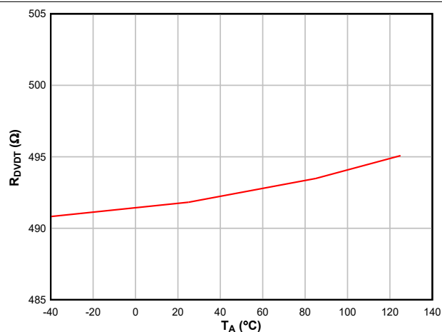
图 6-17. 整个温度范围内的 DVDVT 放电电阻
