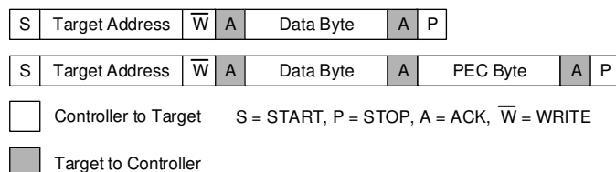
图 7-8. 发送字节
