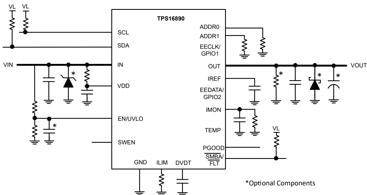
图 8-12. 帶有可选保护元件的电路实现
