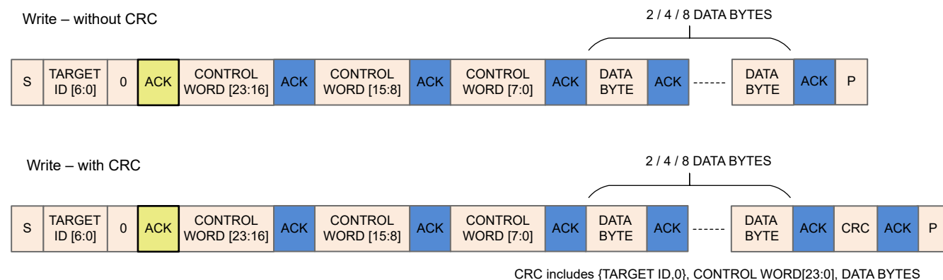
图 6-54. I 2 C 写入事务序列
