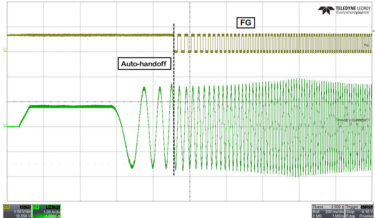
图 9-7. 自动转换
