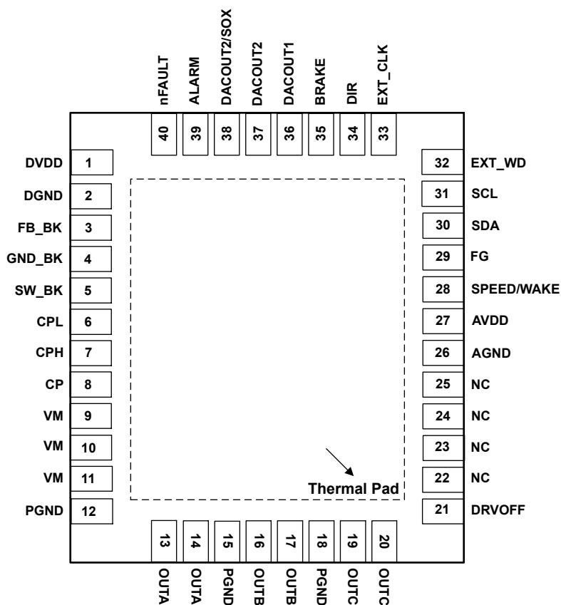
图 4-1. MCF8315C-Q1, 40 引脚 RGF VQFN (带有外露散热焊盘), 顶视图
