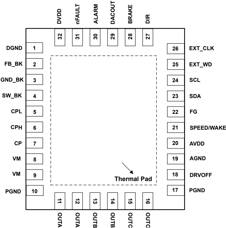
图 4-2. MCF8315C-Q1，32 引脚 RRY WQFN ( 带有外露散热焊盘 )，顶视图
