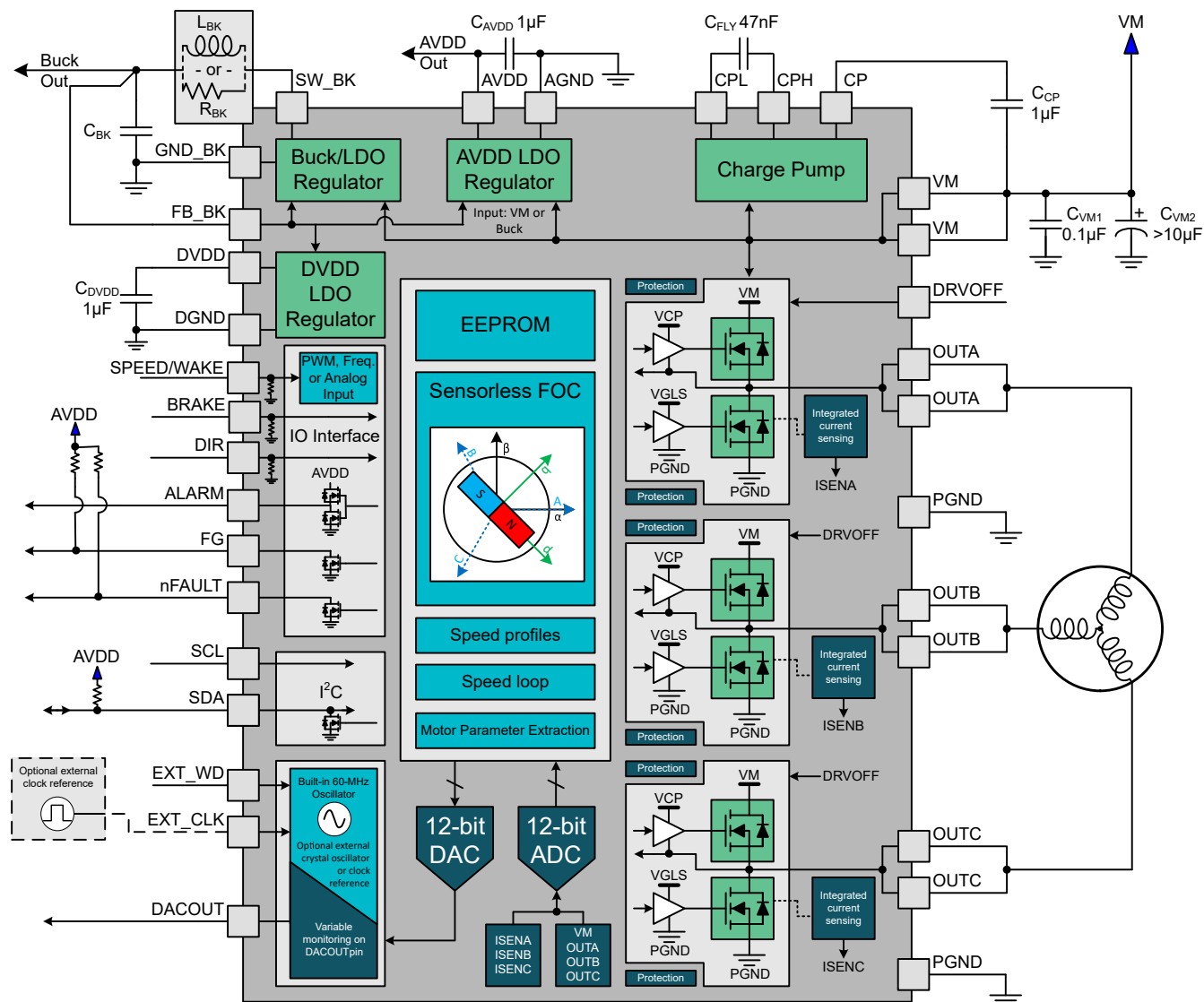
图 6-2. MCF8315C-Q1 (RYY) 功能方框图
