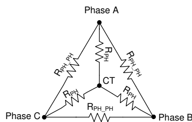
图 6-38. 电机电阻
