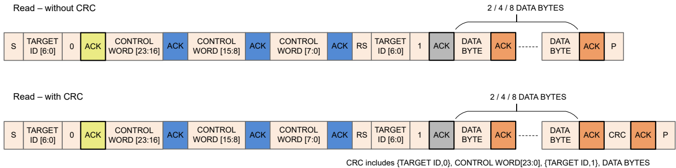
图 6-55. I 2 C 读取事务序列
