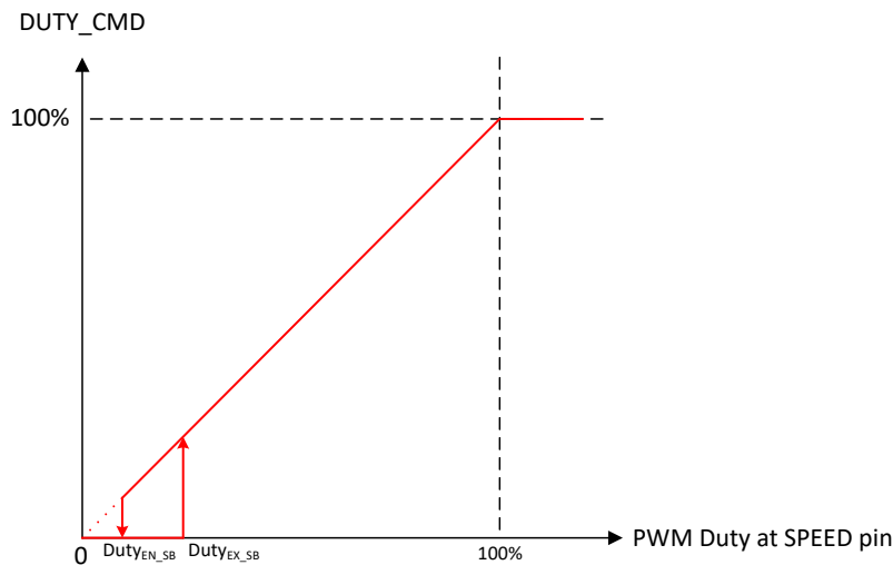
图 6-16. PWM 模式速度控制
