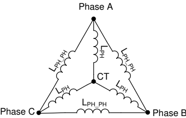
图 6-39. 电机电感
