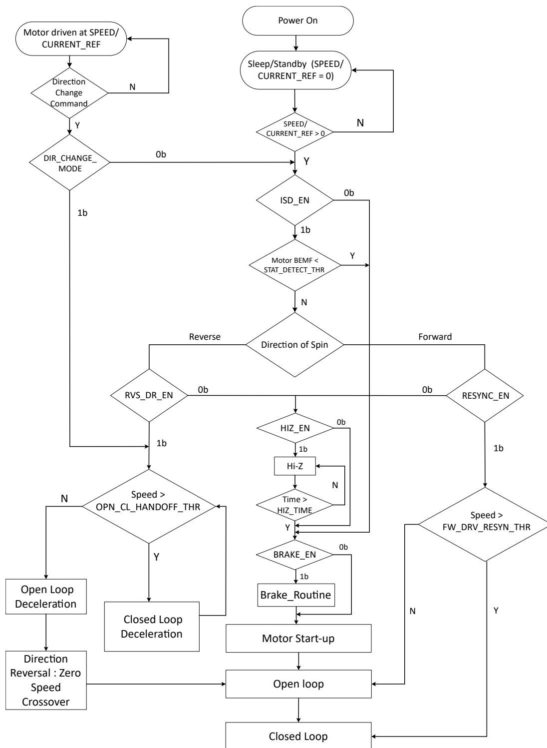
图 6-23. 电机启动序列
