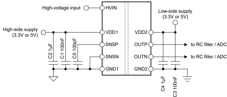
图 8-5. AMC0380D-Q1 去耦
