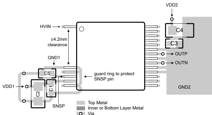
图 8-7. AMC0380D-Q1 ( DFJ 封装 ) 的建议布局
