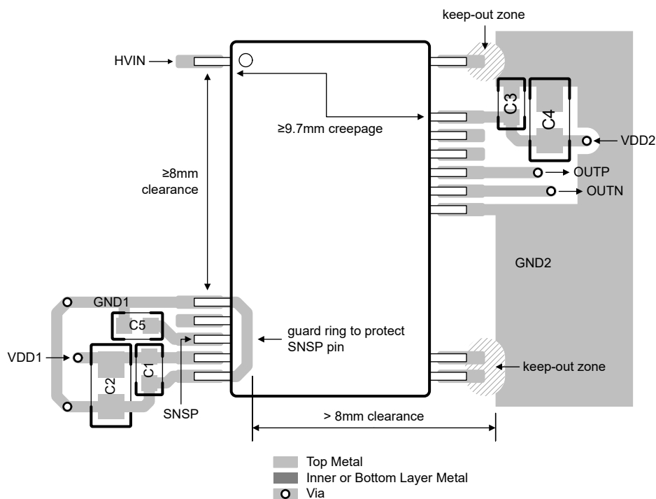
图 8-6. AMC0380D-Q1 ( DFX 封装 ) 的建议布局
