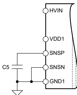
图 8-2. 输入滤波器
