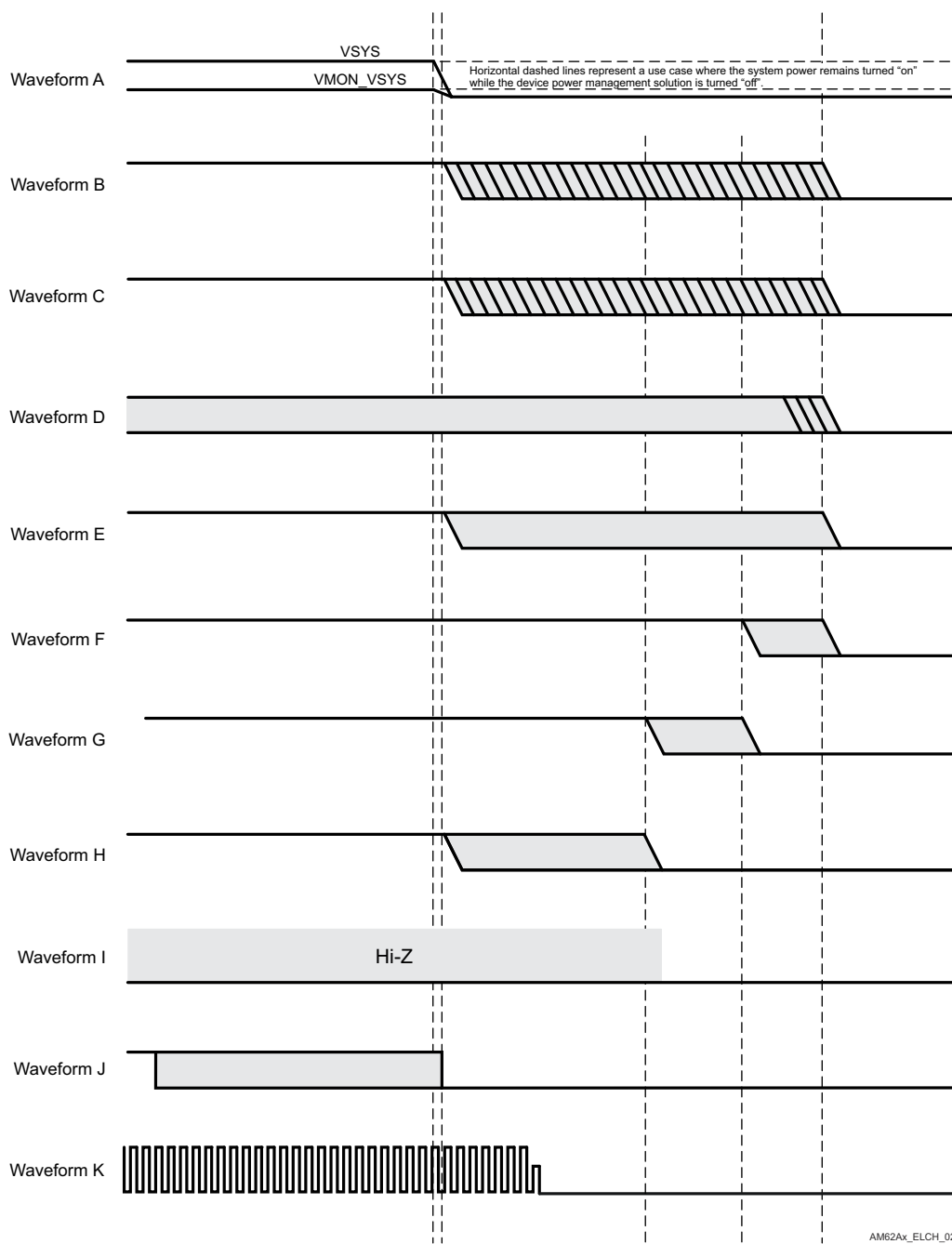
图 6-6. 断电序列
