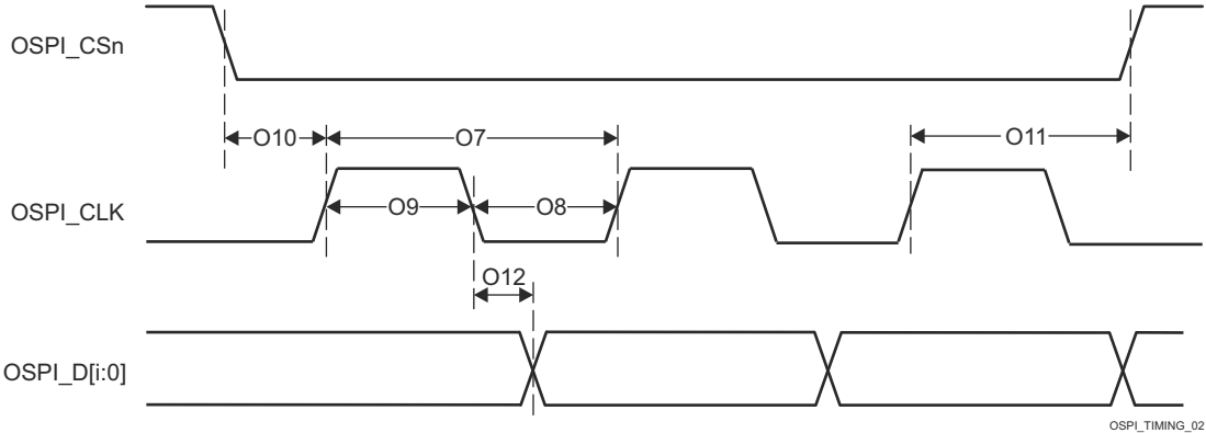
图 6-92. OSPI0 开关特性 - PHY SDR 数据训练
