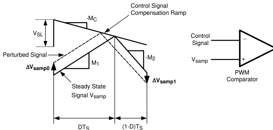
图 6-4. 补偿斜坡可避免次谐波振荡
