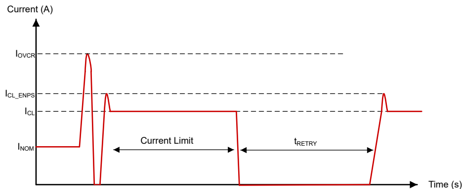
图 7-11. 热短路事件 (自动重试版本)
