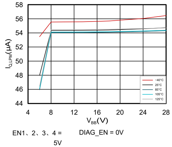
图 6-8. 启用 4 个通道时, 不同温度条件下 I_{Q,LPM} 与 V_{BB} 间的关系
