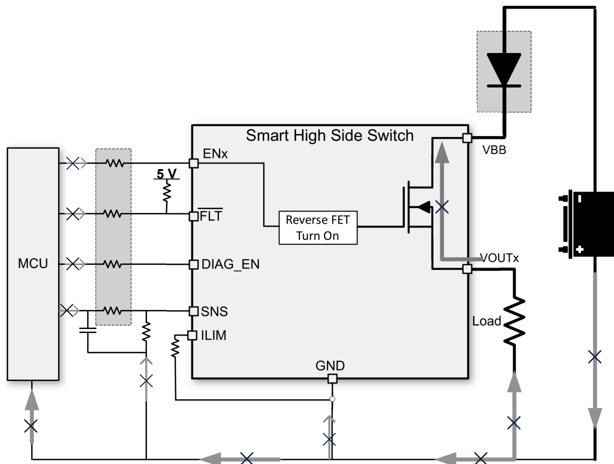
图 7-23. 采用阻断二极管实现反向保护
