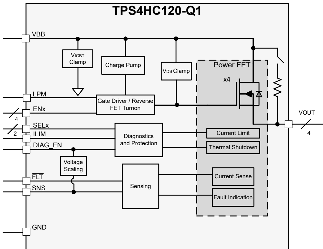
图 7-1. 功能方框图
