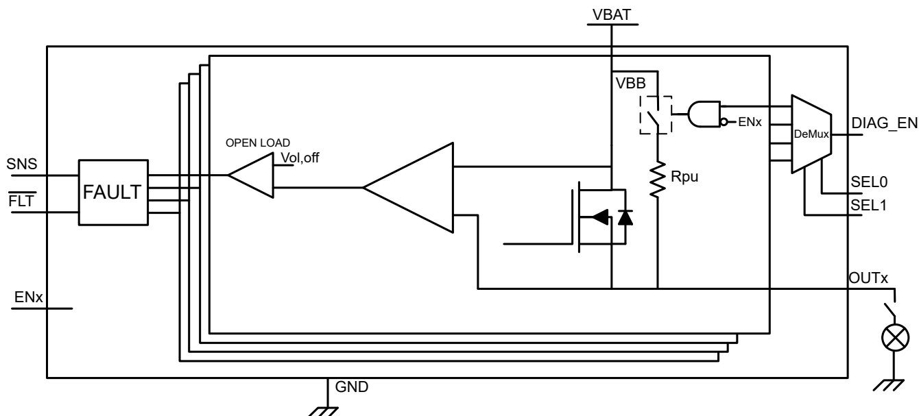
图 7-17. 关断状态下提供开路负载检测
