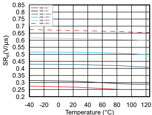
图 6-13. 在 V_{BB} 电压范围内 SR_R 与温度间的关系
