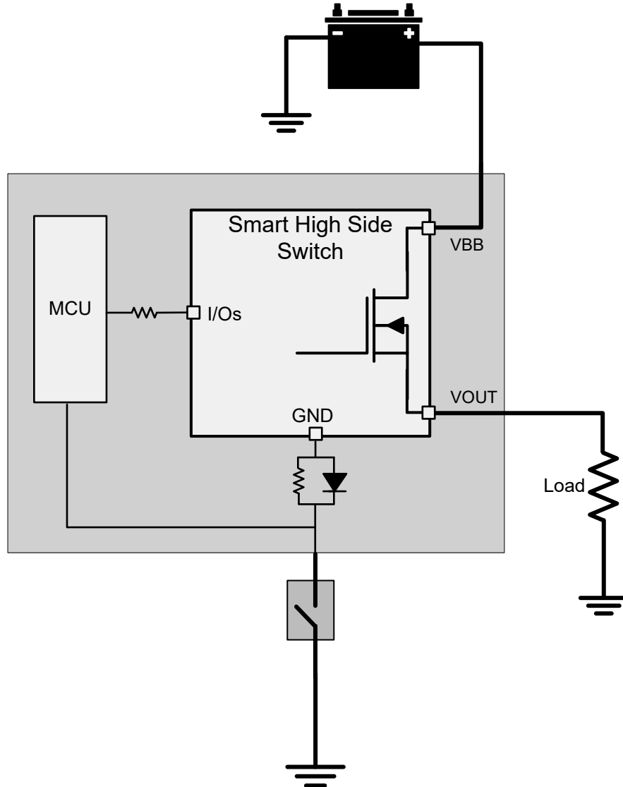
图 7-21. 模块接地失效
