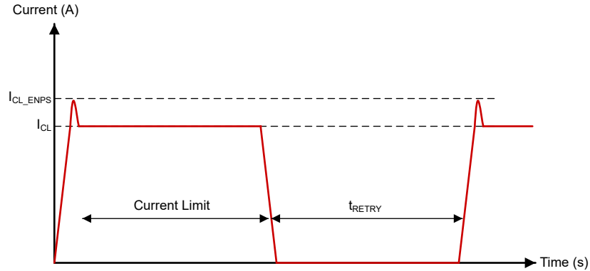
图 7-9. 启用至短路电流限制 (自动重试版本)
