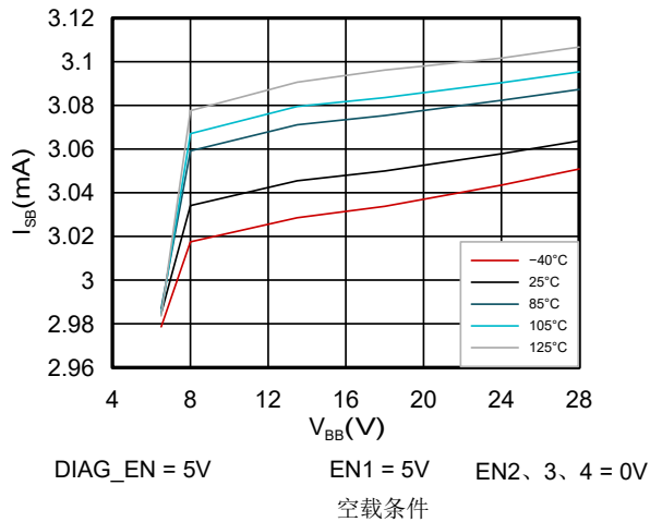
图 6-9. 不同温度条件下 I_{SB} 与 V_{BB} 间的关系
