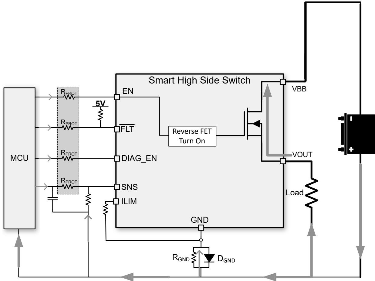
图 7-25. MCU I/O 保护
