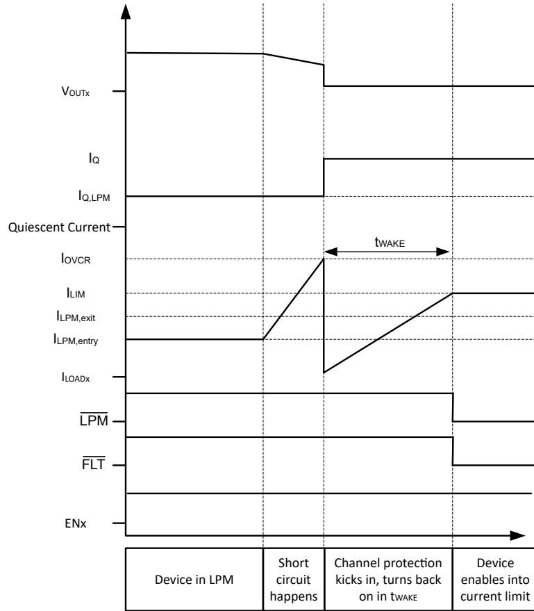
图 7-6. 负载电流快速增加 ( 短路 ) 时退出 LPM
