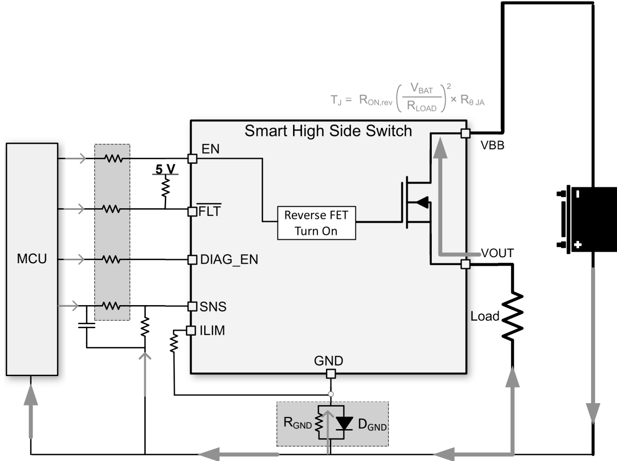
图 7-24. 通过接地网络实现反向保护
