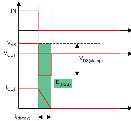
图 7-13. 电感负载关断图
