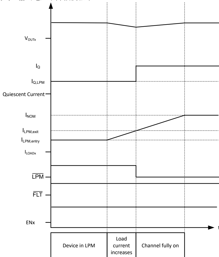
图 7-5. 负载电流缓慢增加时退出 LPM
