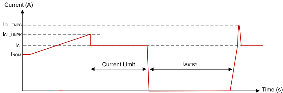
图 7-10. 软短路的线性峰值 (自动重试版本)
