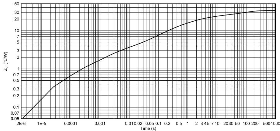
图 8-4. 瞬态热阻抗 (结至环境), T_A = 105^\circ\text{C} , JEDEC 标准 2s2p PCB 布局 (带散热过孔)
