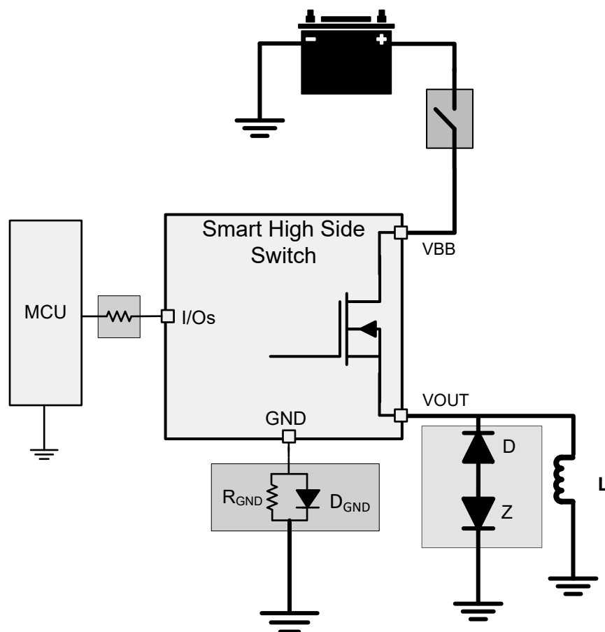
图 7-22. 电池丢失
