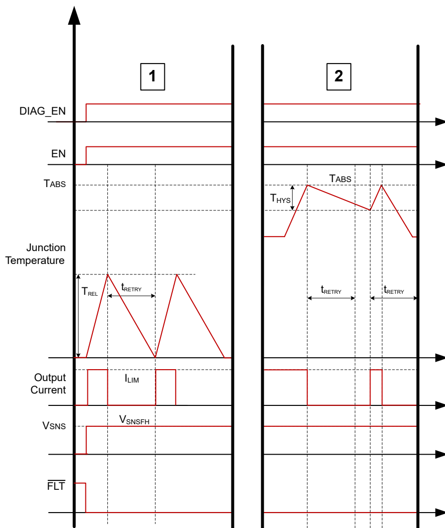
图 7-19. 自动重试版本的热行为
