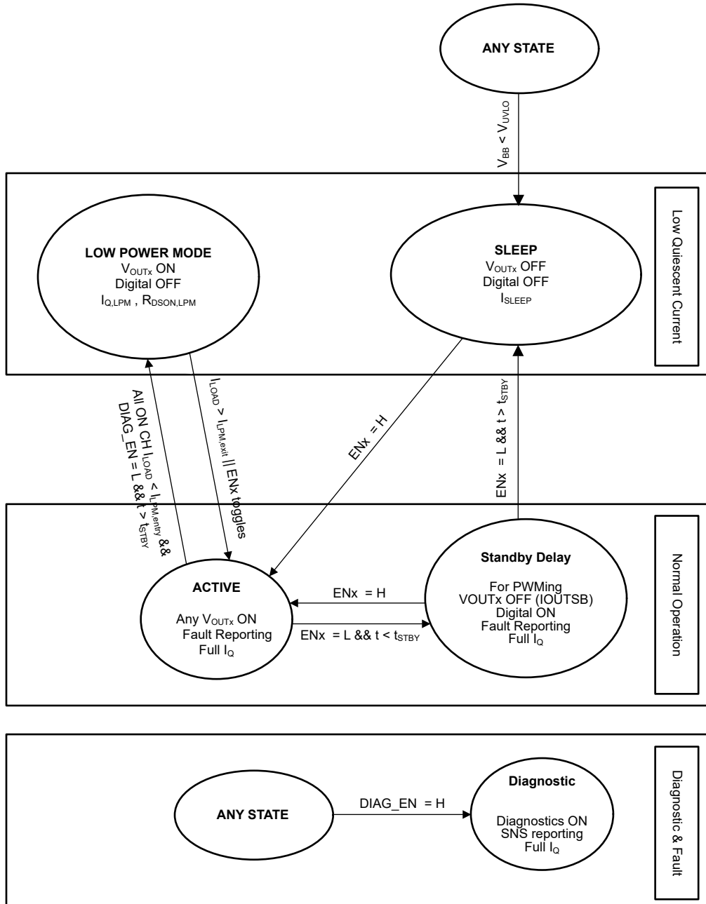
图 7-26. 状态图
