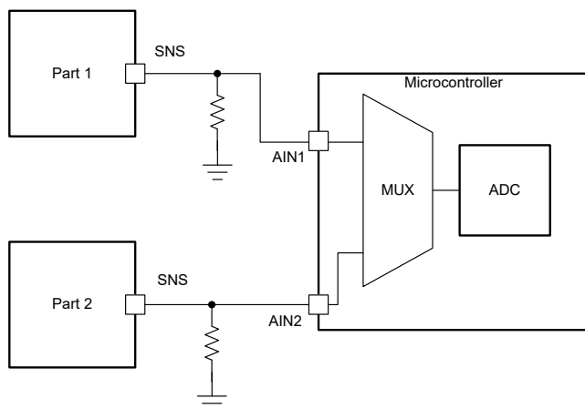
图 7-15. 跨多个器件共享 SNS 方法 1
