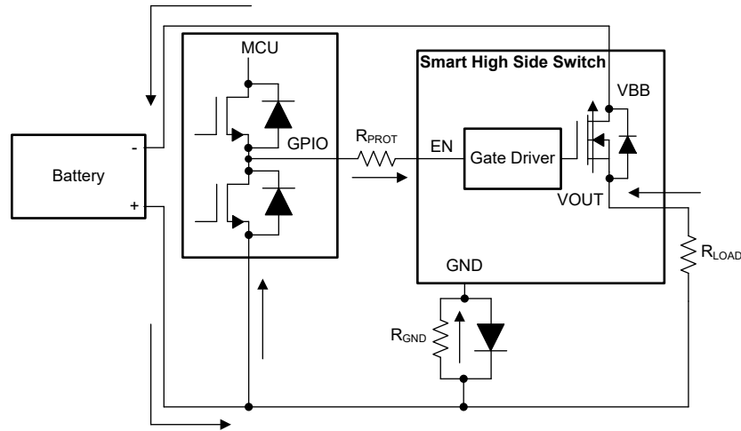
图 7-18. 电池反向电路
