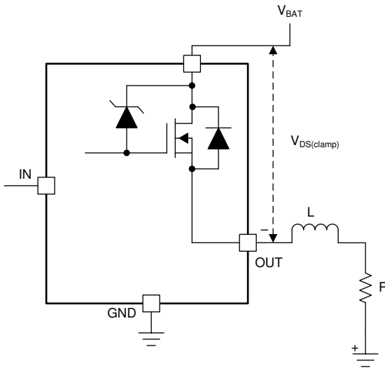
图 7-12. 漏源钳位结构
