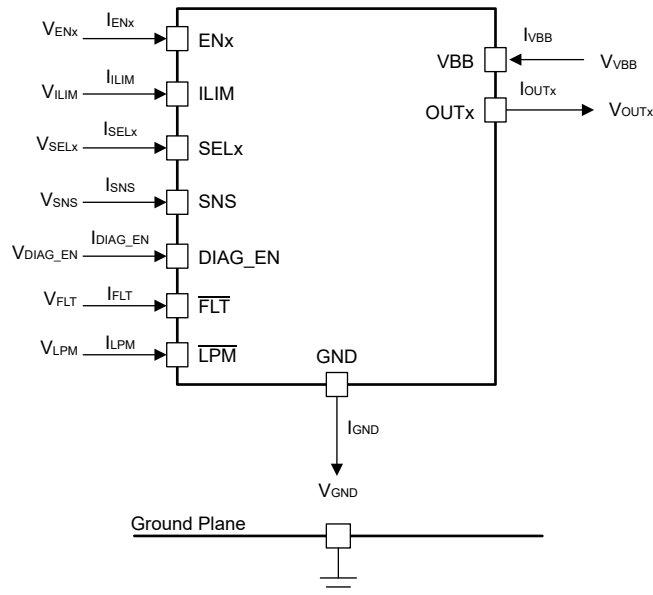
图 7-3. 电压和电流约定
