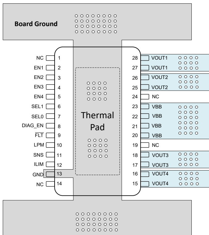
图 8-5. 无接地网络的布局示例
