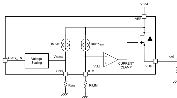
图 7-8. 电流检测和电流限制方框图
