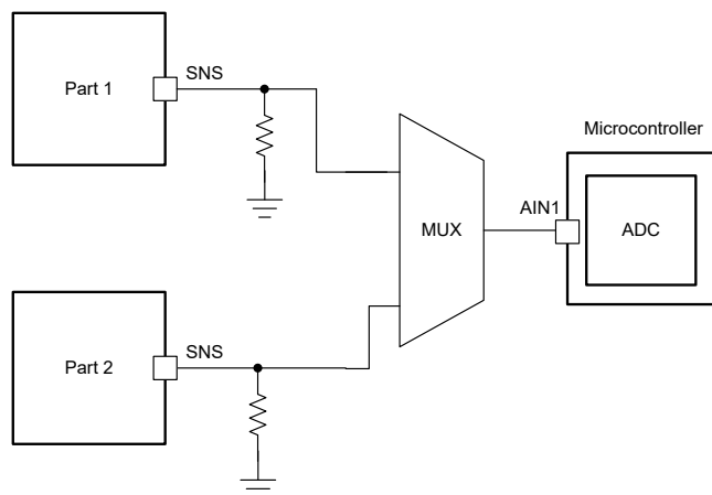
图 7-16. 跨多个器件共享 SNS 方法 2
