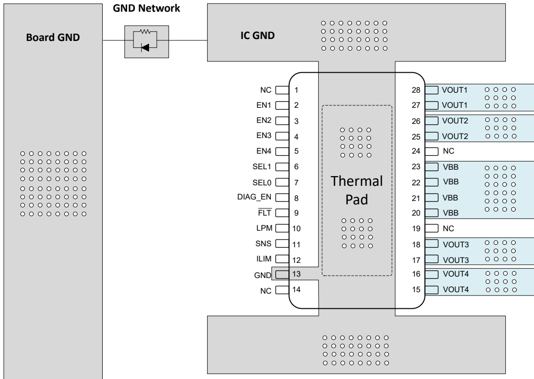
图 8-6. 有接地网络的布局示例
