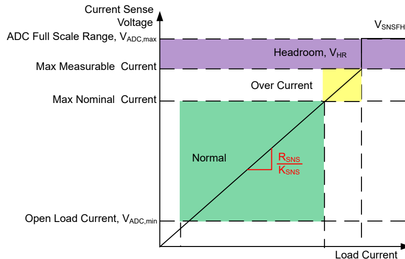
图 7-7. 电流检测引脚上的电压指示
