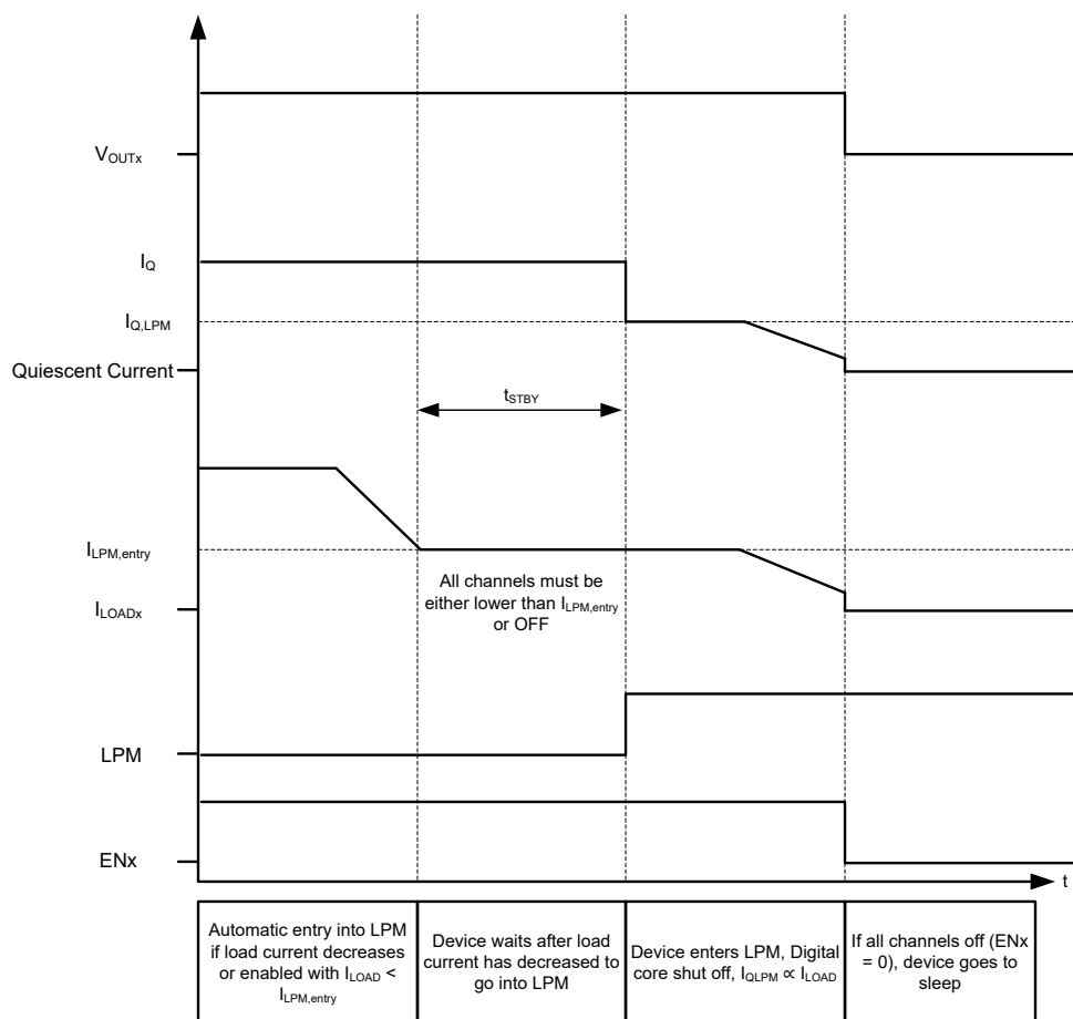
图 7-4. 进入 LPM
