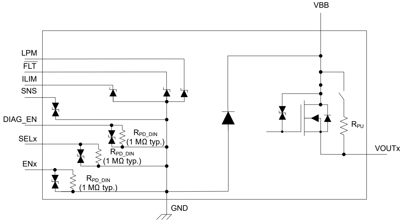
图 7-2. 内部二极管图
