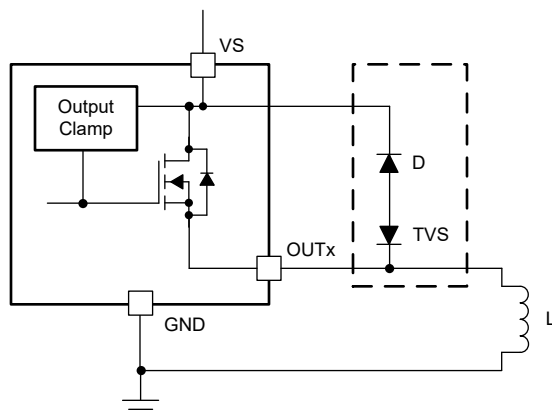
图 7-14. 通过外部电路提供保护
