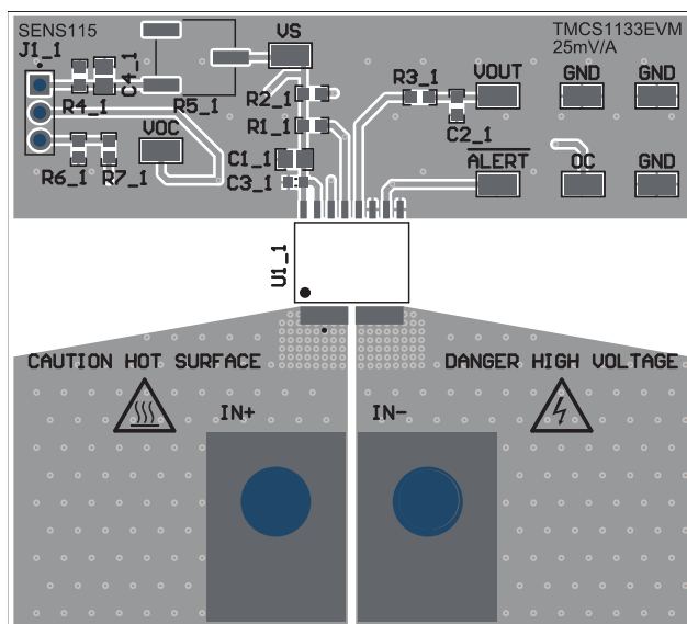
图 9-6. 建议的电路板布局布线
