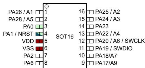
图 6-4. 16 引脚 DYY (SOT) (顶视图)
