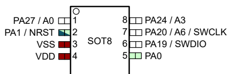
图 6-5. 8 引脚 DDF (SOT) (顶视图)
