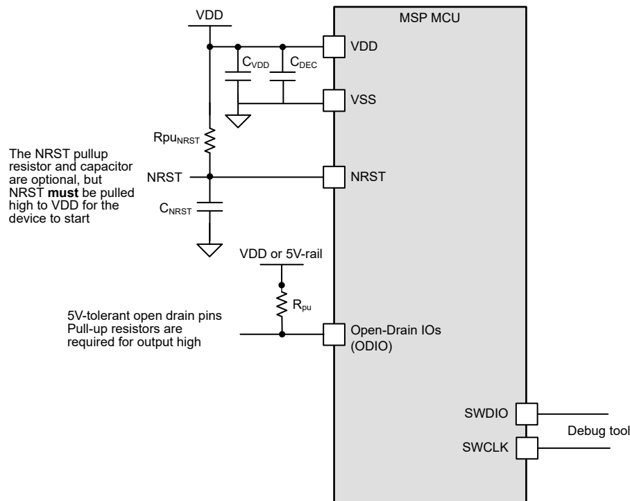
图 9-1. 典型应用原理图
