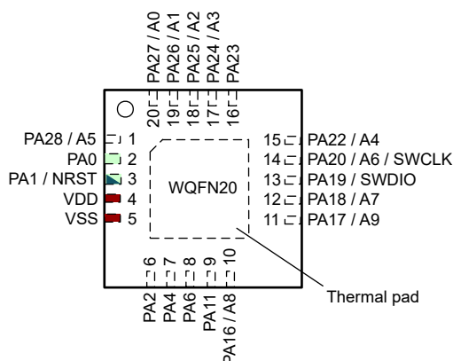
图 6-3. 20 引脚 RUK (WQFN) (顶视图)
