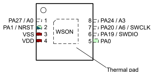
图 6-6. 8 引脚 DSG (WSON) (顶视图)
