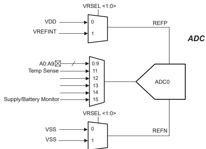
图 8-2. 模拟连接
