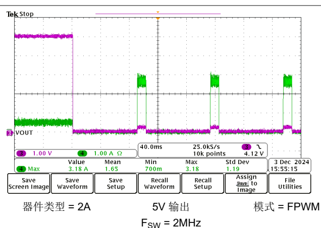
图 8-21. 应用短路
