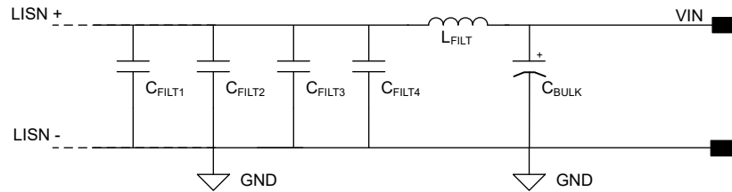
图 8-34. 典型输入 EMI 滤波器原理图
