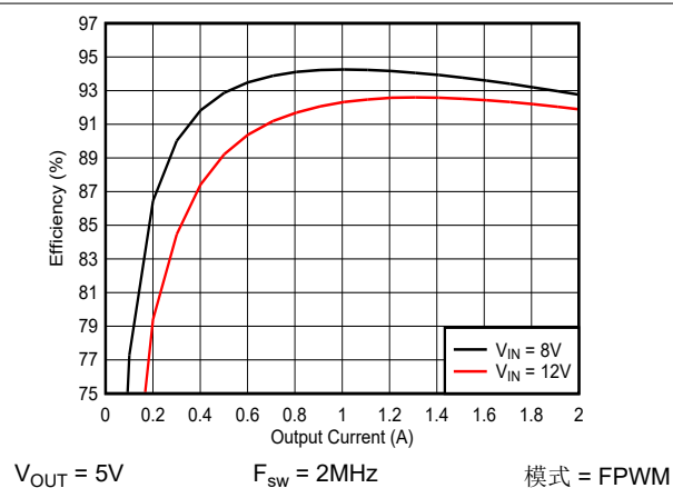
图 8-7. 效率
