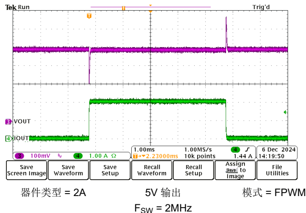
图 8-15. 0A 至 2A 负载瞬态
