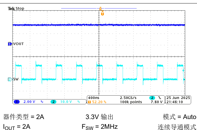
图 8-23. 稳态波形
