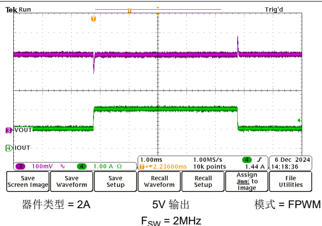
图 8-16. 1A 至 2A 负载瞬态
