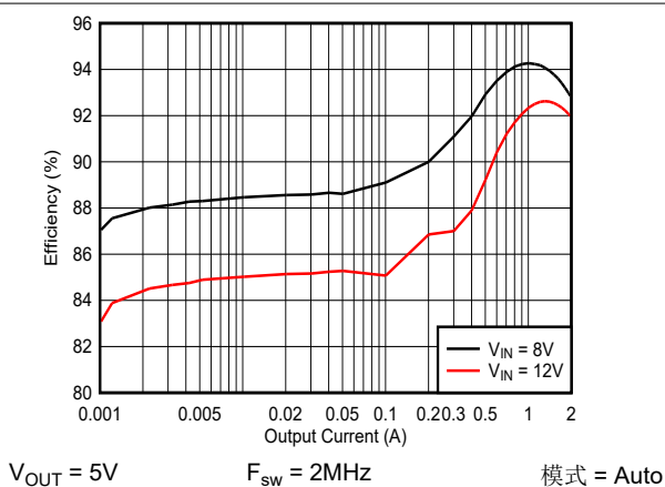
图 8-6. 效率
