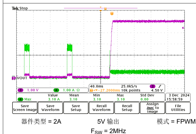
图 8-22. 短路恢复
