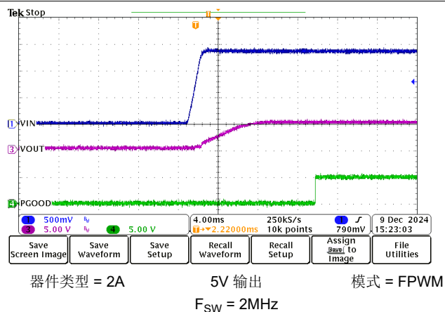
图 8-19. 启动运行
