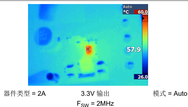
图 8-25. 热性能
