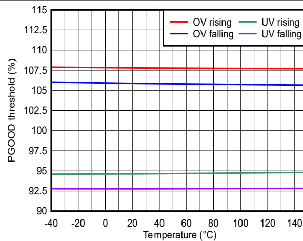
图 6-11. PGOOD 阈值
