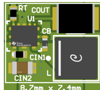
EVM 布局 - 2.2MHz 3.3V 固定输出
