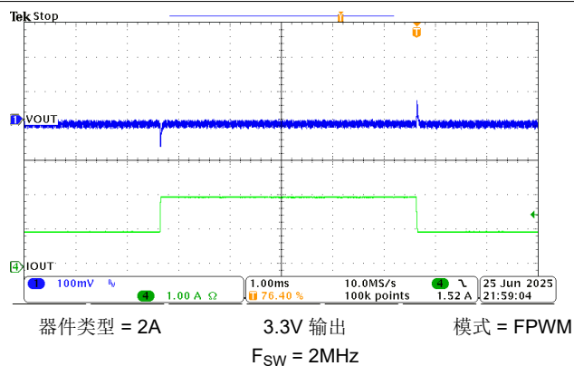
图 8-18. 1A 至 2A 负载瞬态
