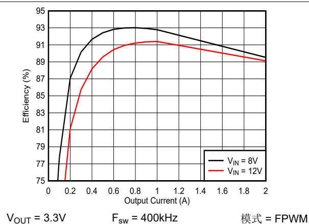
图 8-5. 效率
