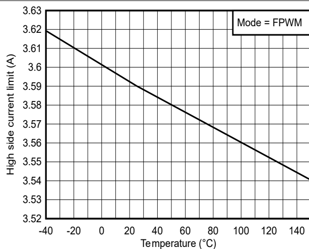
图 6-1. 高侧 MOSFET 电流限制
