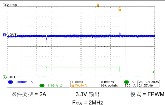
图 8-17. 0A 至 1A 负载瞬态
