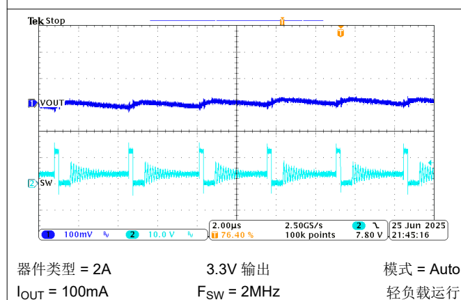
图 8-24. 稳态波形
