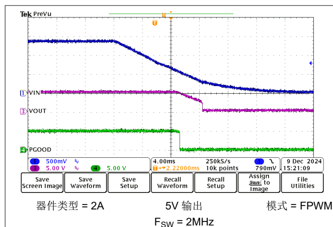
图 8-20. 关断操作
