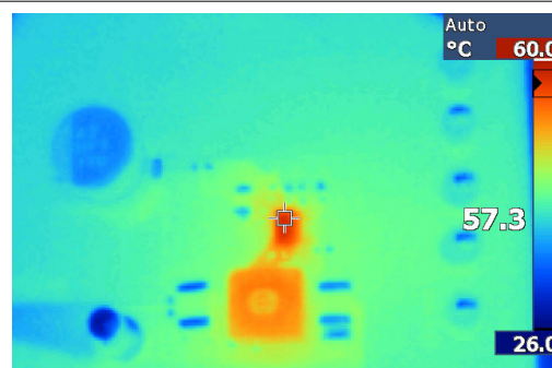
图 8-23. 热性能
