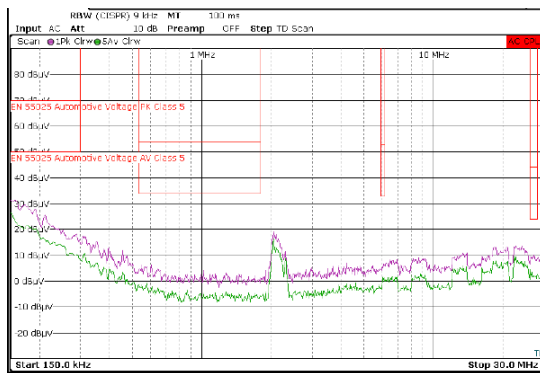
图 8-26. 传导 EMI 与 CISPR25 限值 (紫色：峰值信号，绿色：平均信号)，LMR60440QEVm
