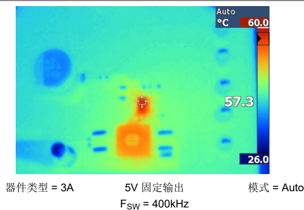
图 8-25. 热性能
