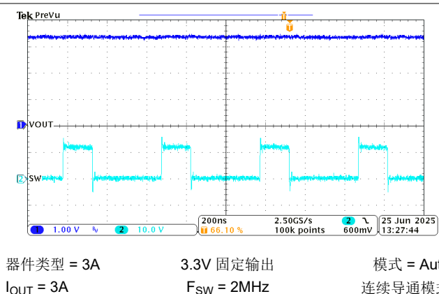
图 8-21. 稳态波形
