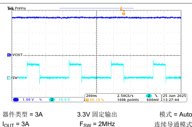
图 8-21. 稳态波形
