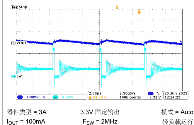
图 8-22. 稳态波形
