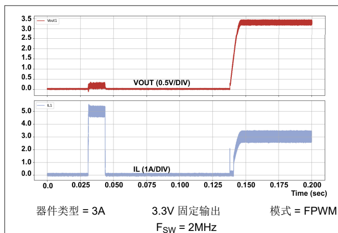
图 8-20. 短路恢复
