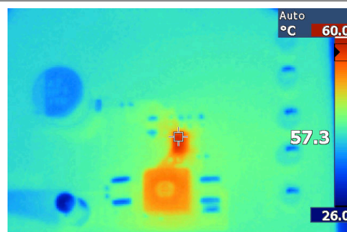
图 8-23. 热性能
