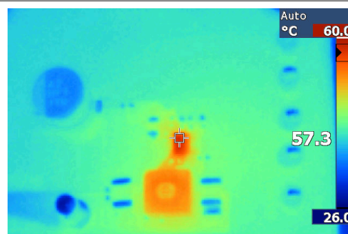
图 8-23. 热性能
