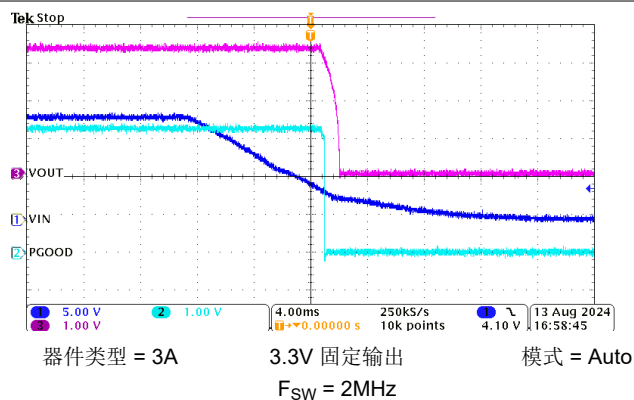
图 8-18. 关断操作
