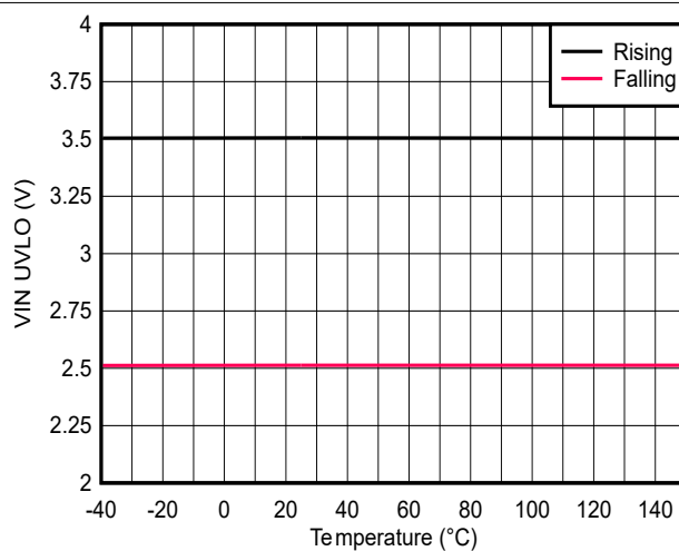
图 6-10. 输入电压 UVLO - B 型号
