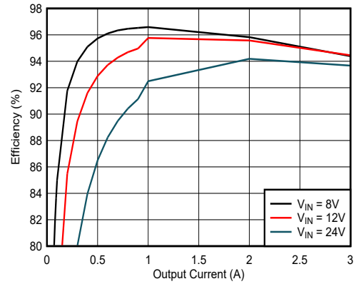
图 8-9. 效率
