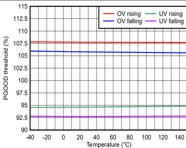
图 6-11. PGOOD 阈值
