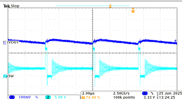
图 8-20. 短路恢复
