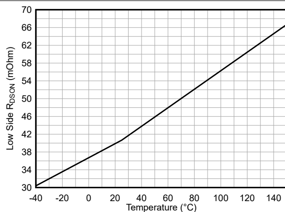
图 6-4. 低侧 MOSFET R_{DS-ON}
