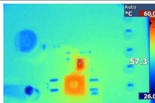
图 8-23. 热性能
