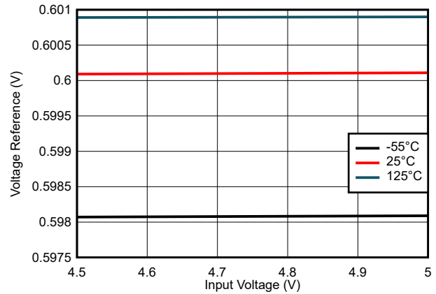
图 6-20. 内部电压基准与输入电压间的关系
