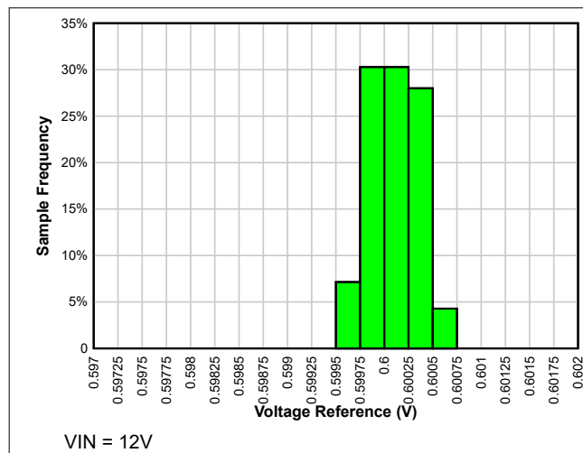
图 6-51. T_A = 25^{\circ}\text{C} 时的电压基准分布
