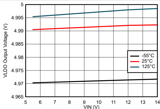
图 6-2. 内部线性稳压器输出电压与输入电压间的关系
