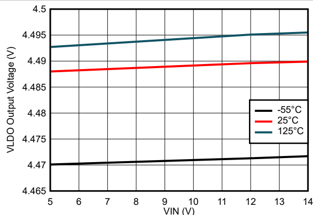
图 6-1. 内部线性稳压器输出电压与输入电压间的关系
