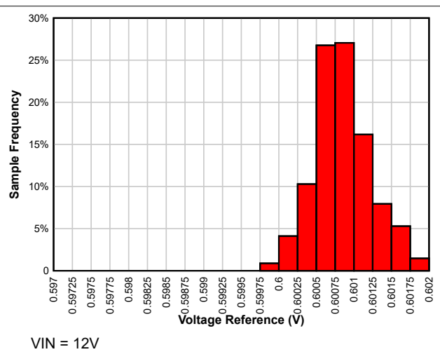
图 6-52. T_A = 125^{\circ}\text{C} 时的电压基准分布
