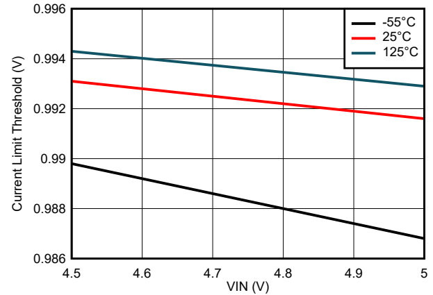
图 6-22. 电流限制阈值与输入电压间的关系
