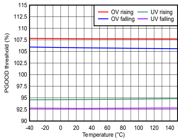
图 6-10. PGOOD 阈值
