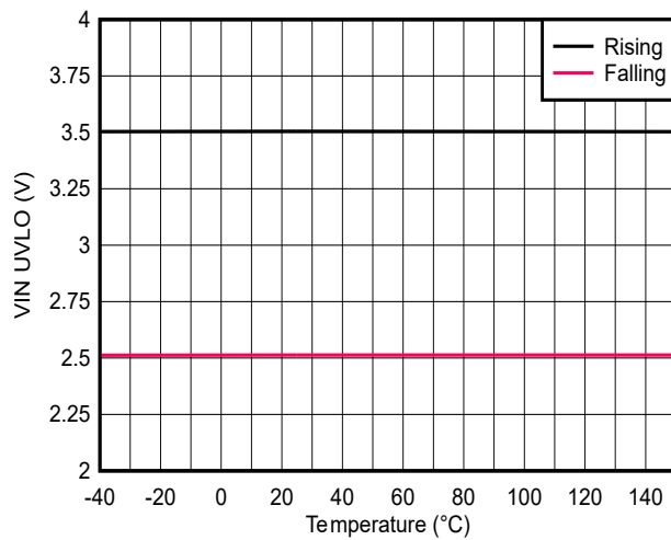
图 6-9. 输入电压 UVLO
