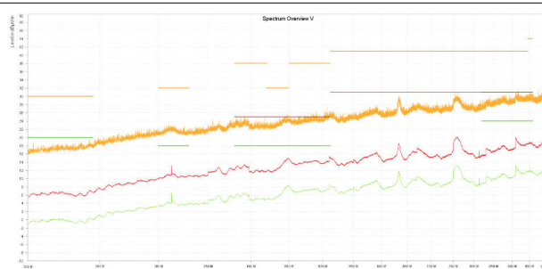
图 8-27. 辐射 EMI 双锥垂直与 CISPR25 限值， LMR60440QEVM
