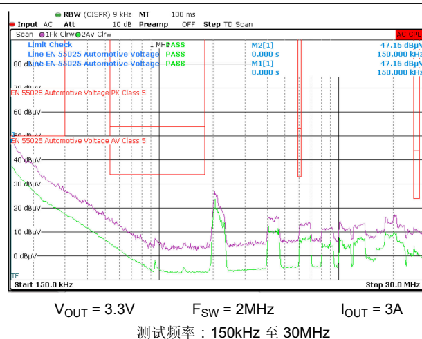
图 8-24. 传导 EMI 与 CISPR25 限值 (紫色: 峰值信号, 绿色: 平均信号), LMR60440QEVm
