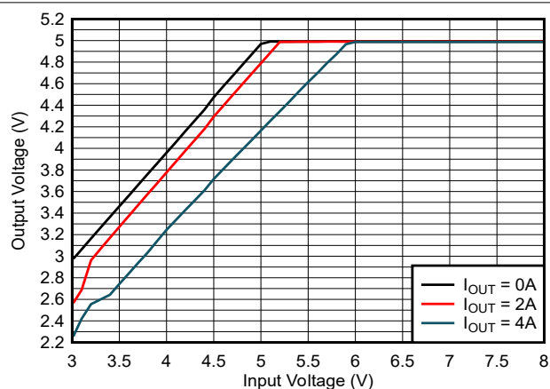
图 8-12. 压降
