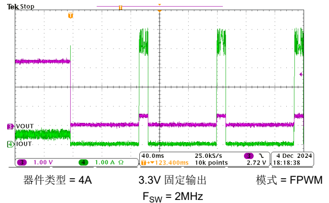
图 8-21. 应用短路
