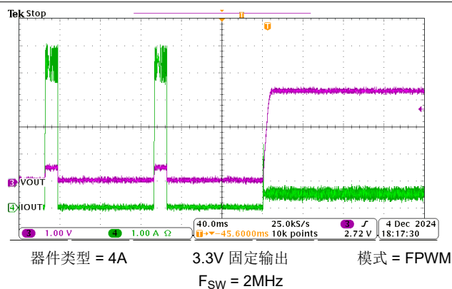
图 8-22. 短路恢复
