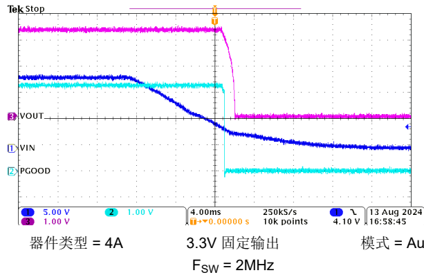
图 8-20. 关断操作
