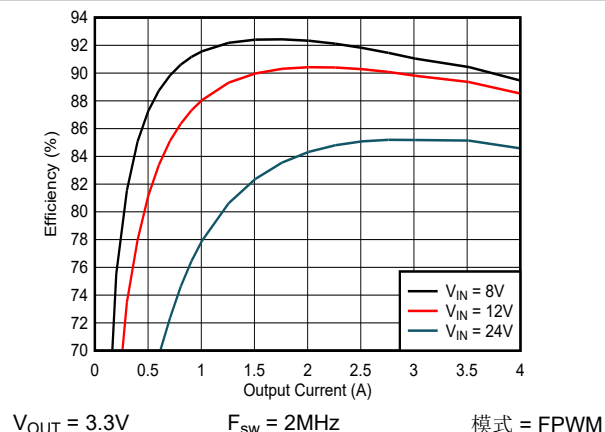
图 8-3. 效率
