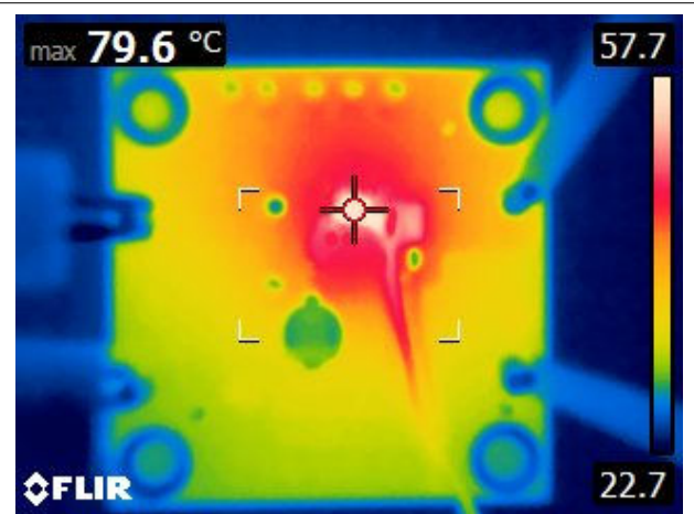
图 8-21. 应用短路
