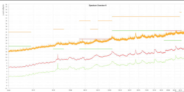
图 8-28. 辐射 EMI 双锥水平与 CISPR25 限值， LMR60440QEVM
