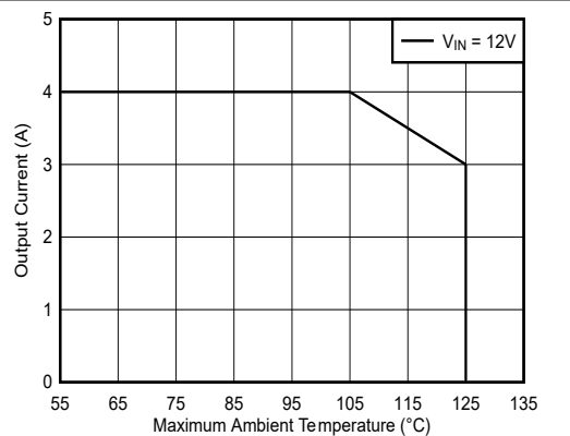
图 8-15. 输出电流与最大环境温度间的关系
