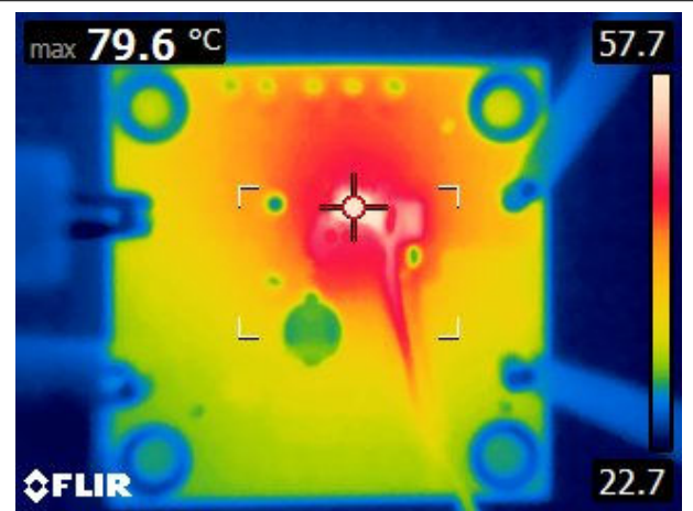
图 8-21. 应用短路
