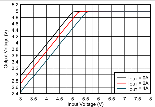
图 8-11. 压降
