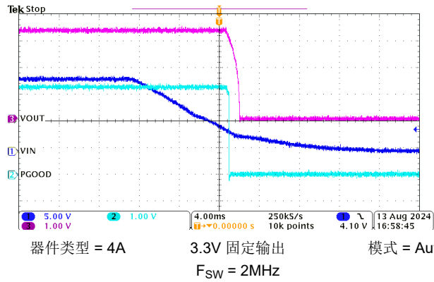
图 8-20. 关断操作
