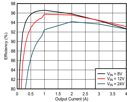
图 8-9. 效率
